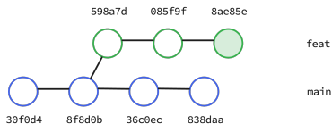
Figura: Log dei commit prima di un merge
