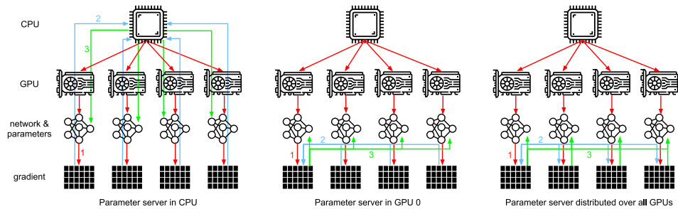
Figure 13.7.3 Parameter synchronization strategies.
