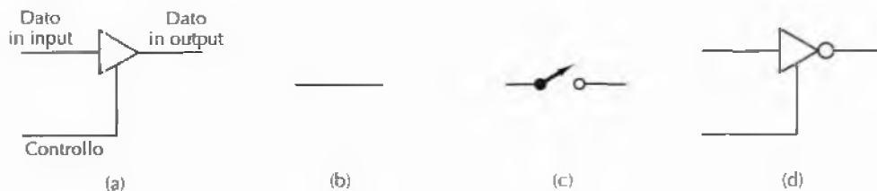
Figura 3.30 (a) Buffer non invertente. (b) Risultato di (a) quando il controllo è alto. (c) Risultato di (a) quando il controllo è basso. (d) Buffer invertente.
