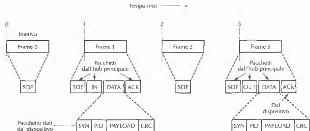
Figura 3.59 L'hub principale USB spedisce frame ogni millisecondo.
