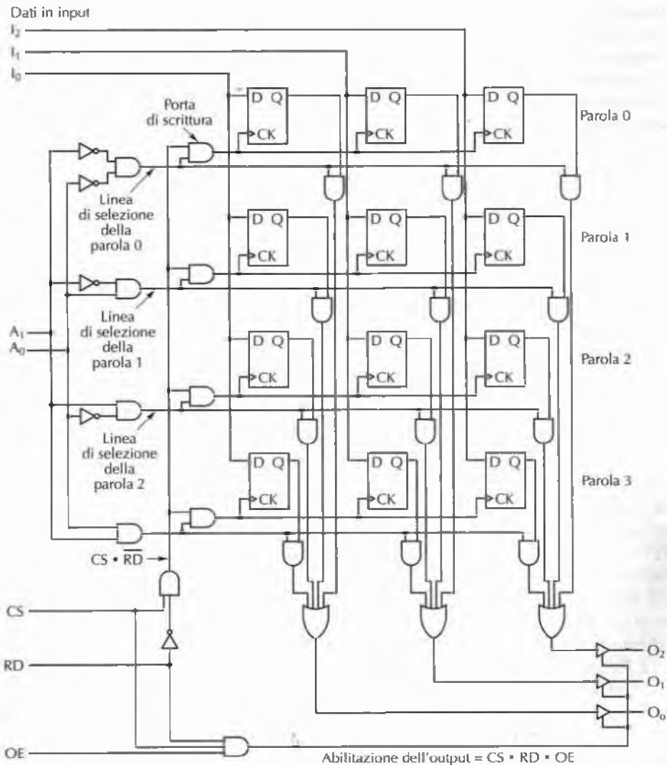
Figura 3.29 Diagramma logico di una memoria 4 x 3. Ogni riga è una delle quattro parole a 3 bit. Lettura e scrittura riguardano sempre parole complete.
