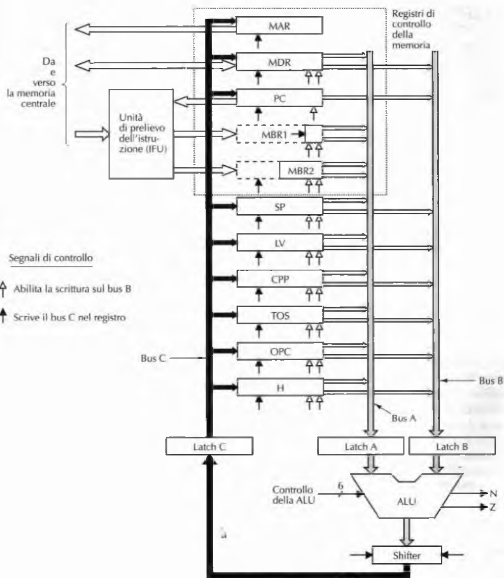
Figura 4.31 Percorso dati a tre bus utilizzato in Mic-3.
