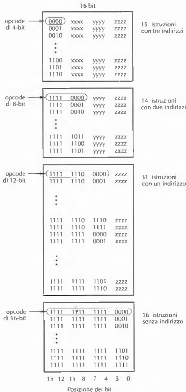
Figura 5.13 Un opcode espandibile che consente di avere 15 istruzioni con tre indirizzi, 14 con due indirizzi, 31 con un indirizzo e 16 senza indirizzo. I campi contrassegnati con xxxx, yyyy e zzzz sono di 4 bit.
