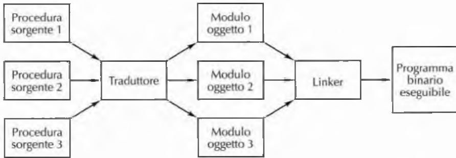
Figura 7.13 Generazione tramite un linker di un programma eseguibile binario a partire da un gruppo di procedure sorgente tradotte indipendentemente.
