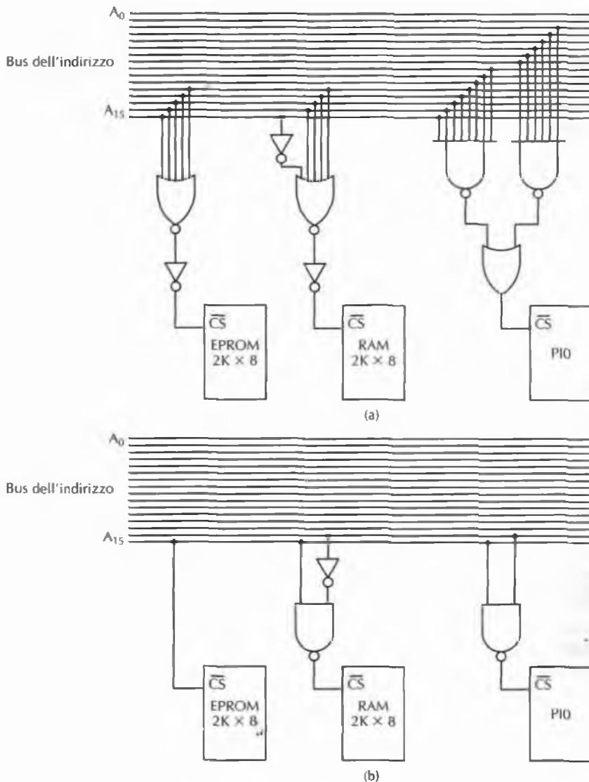
Figura 3.62 Decodifica dell'indirizzo: (a) completa; (b) parziale.
