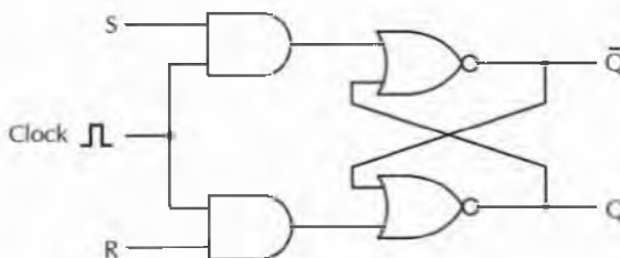
Figura 3.23 Latch SR temporizzato.
