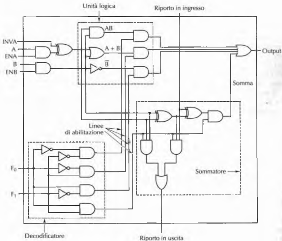
Figura 3.19 ALU a 1 bit.
