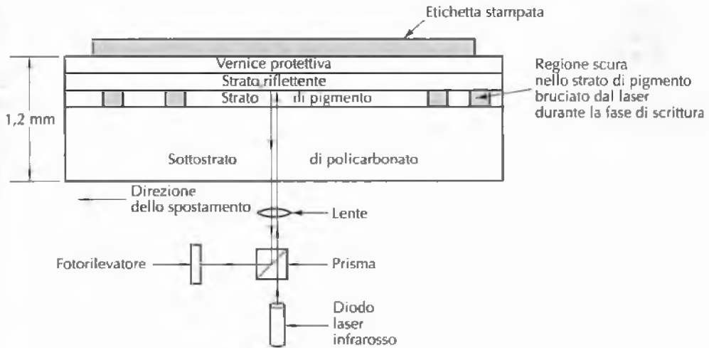
Figura 2.26 Spaccato di un disco CD-R e del laser (non in scala). La struttura di un CD-ROM è simile, fatta eccezione per la mancanza dello strato di pigmento e per la presenza di uno strato di alluminio con pit al posto dello strato riflettente.
