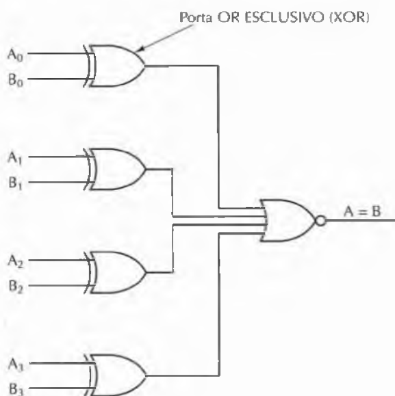
Figura 3.14 Semplice comparatore a 4 bit.
