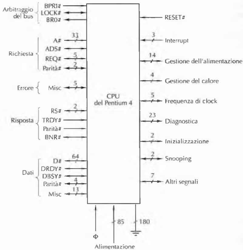
Figura 3.45 Disposizione logica dei contatti del Pentium 4. I nomi interamente in maiuscolo sono i nomi ufficiali di Intel per i singoli segnali; gli altri sono nomi di gruppi di segnali o descrizioni dei segnali.
