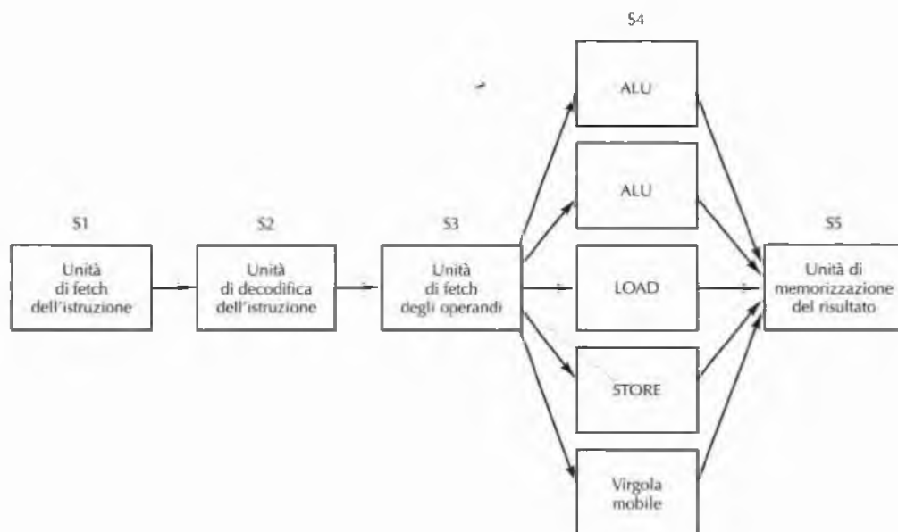
Figura 2.6 Processore superscalare con cinque unità funzionali.
