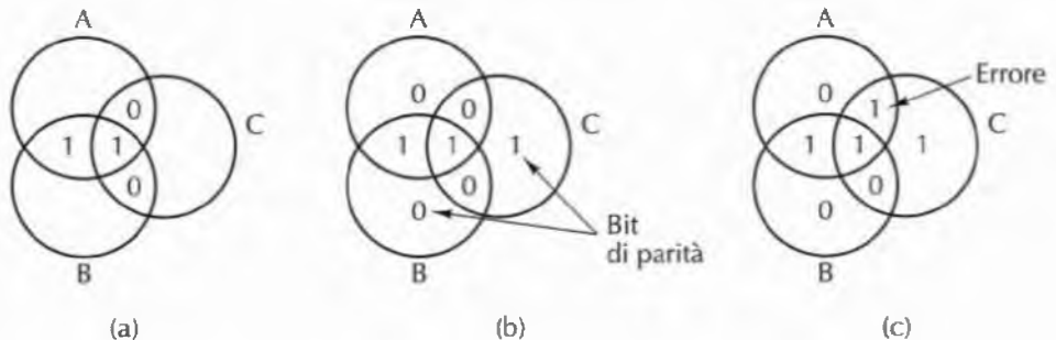
Figura 2.14 (a) Codifica di 1100. (b) Aggiunta della parità pari. (c) Errore in AC .
