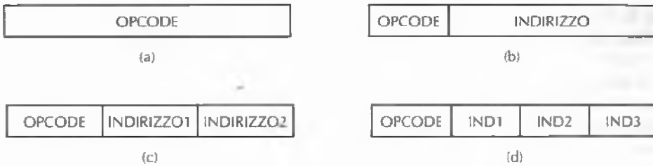
Figura 5.10 Quattro formati d'istruzione: (a) Istruzione senza indirizzi. (b) Istruzione a un indirizzo. (c) Istruzione a due indirizzi. (d) Istruzione a tre indirizzi.
