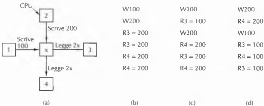
Figura 8.22 (a) Due CPU che scrivono una parola di memoria letta da altre due CPU. (b)-(d) Tre permutazioni dell'ordine temporale delle due scritture e delle quattro letture.
