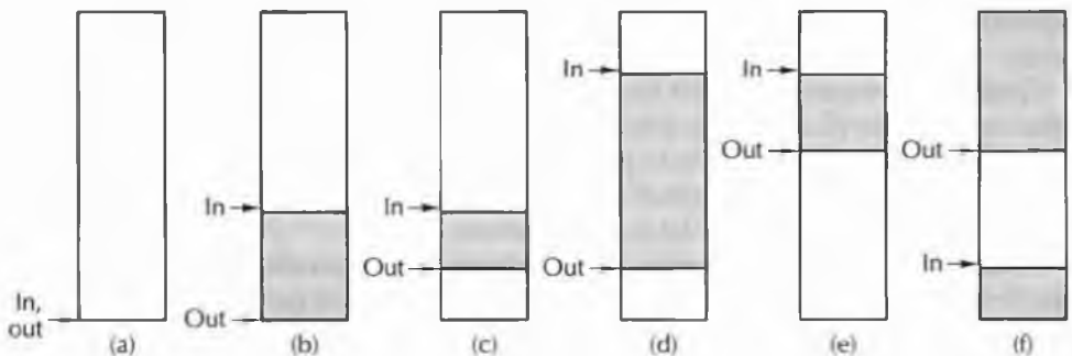
Figura 6.24 Uso di un buffer circolare.
