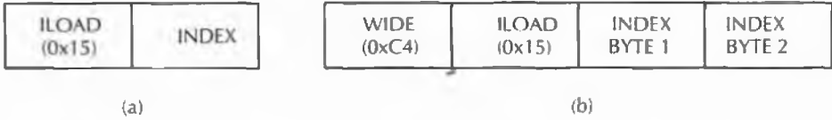
Figura 4.19 (a) ILOAD con un indice a 1 byte. (b) WIDE ILOAD con un indice a 2 byte.
