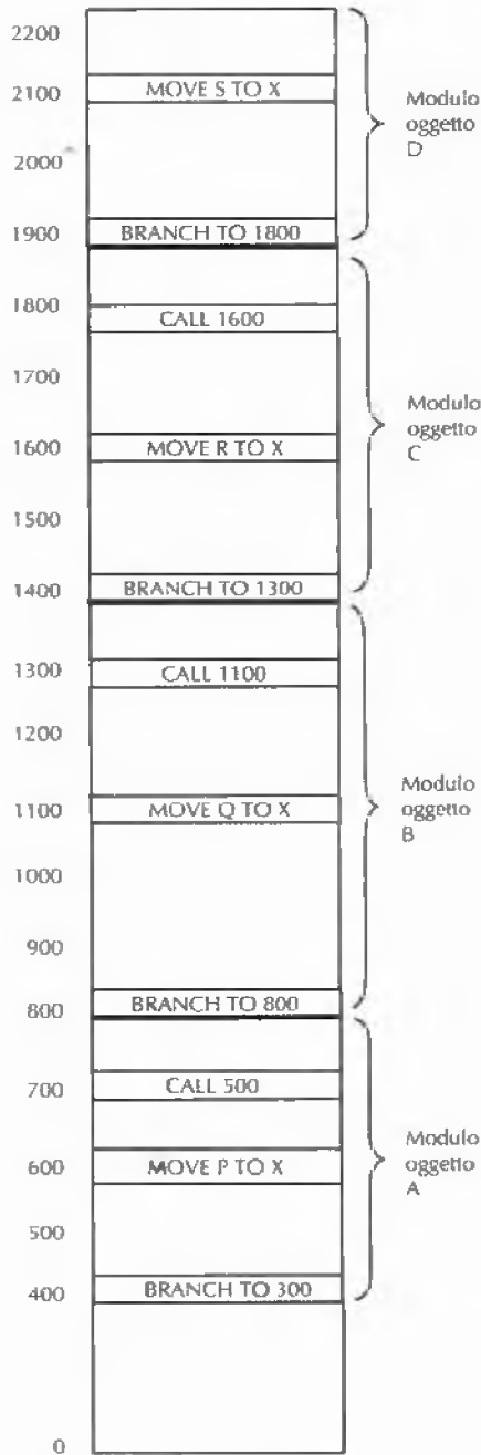
Figura 7.17 Programma binario rilocato della Figura 7.15(b) spostato all'indirizzo 300. Molte istruzioni si riferiscono ora a indirizzi di memoria errati.
