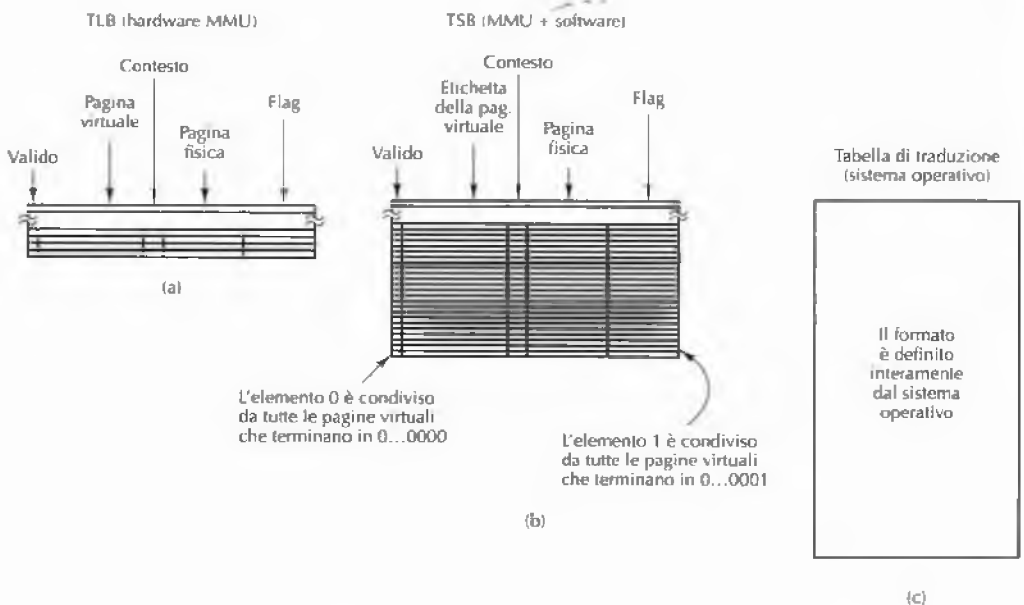
Figura 6.18 Strutture dati per la traduzione d'indirizzi virtuali dell'UltraSPARC. (a) TLB. (b) TSB. (c) Tabella di traduzione.
