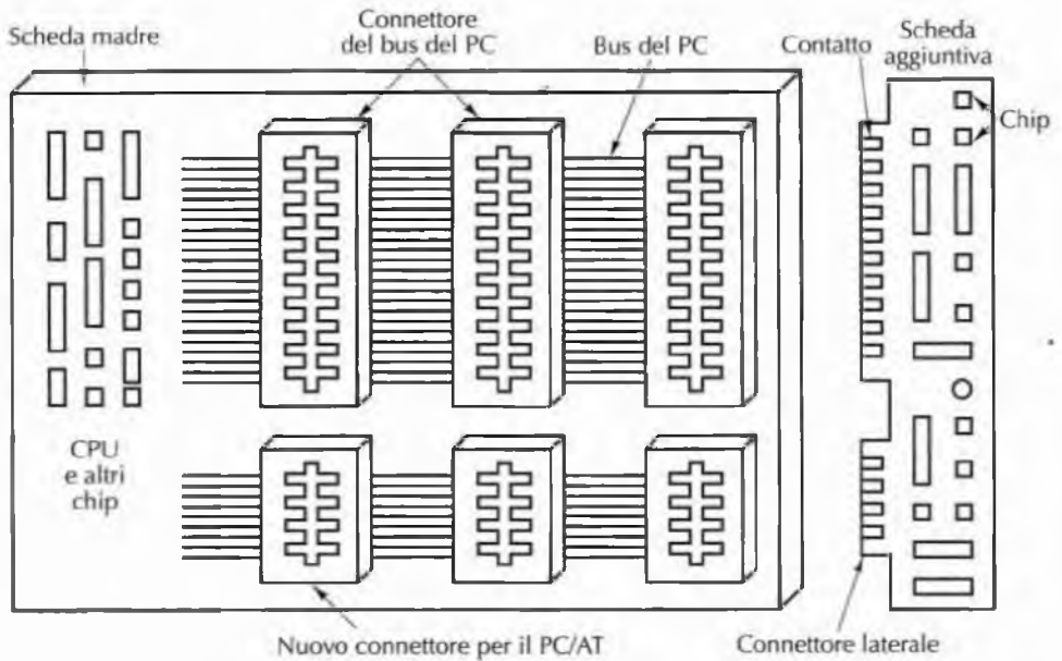
Figura 3.51 I due componenti del bus del PC/AT: una parte uguale a quella del PC originario e una parte nuova.
