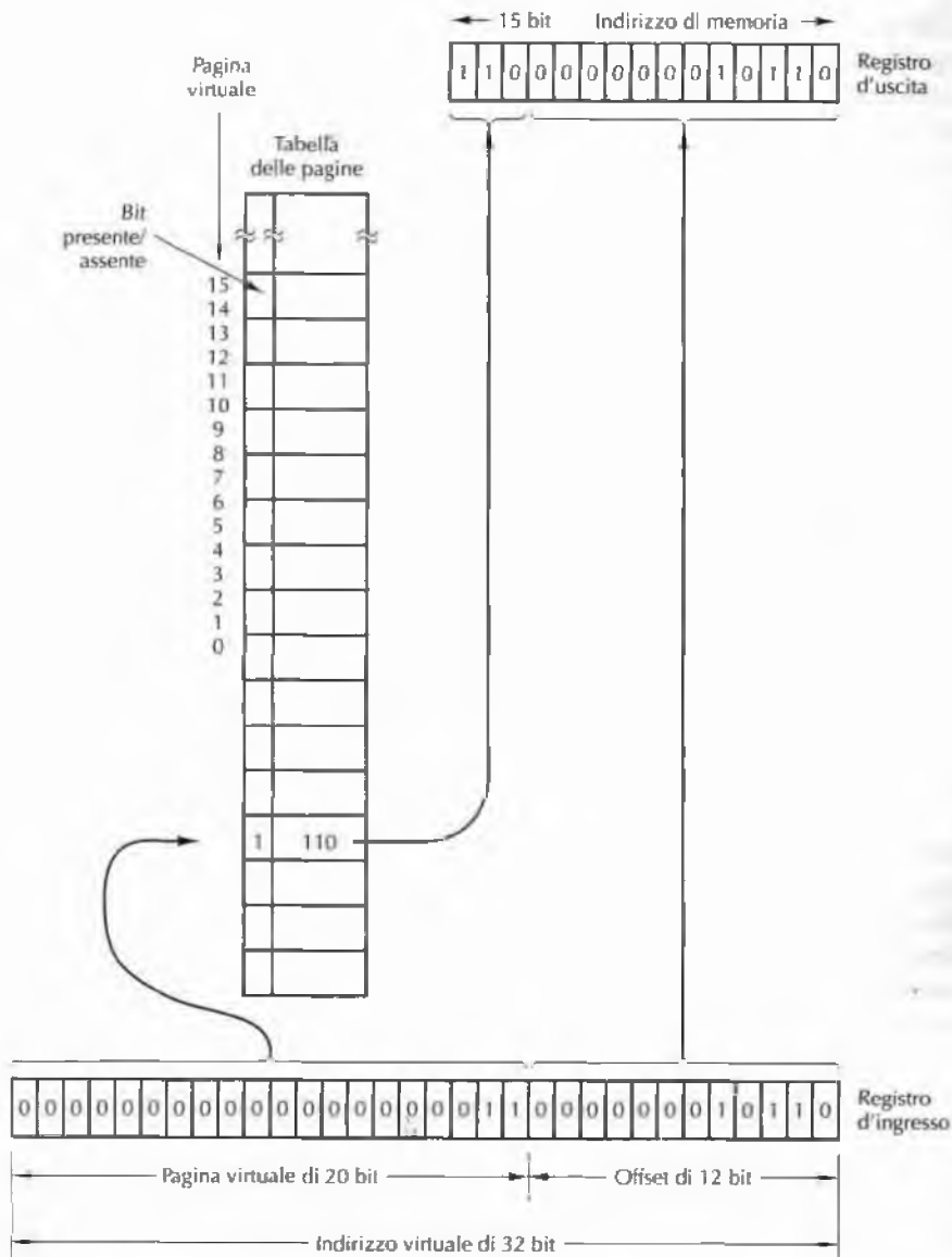
Figura 6.4 Formazione di un indirizzo fisico a partire da un indirizzo virtuale.
