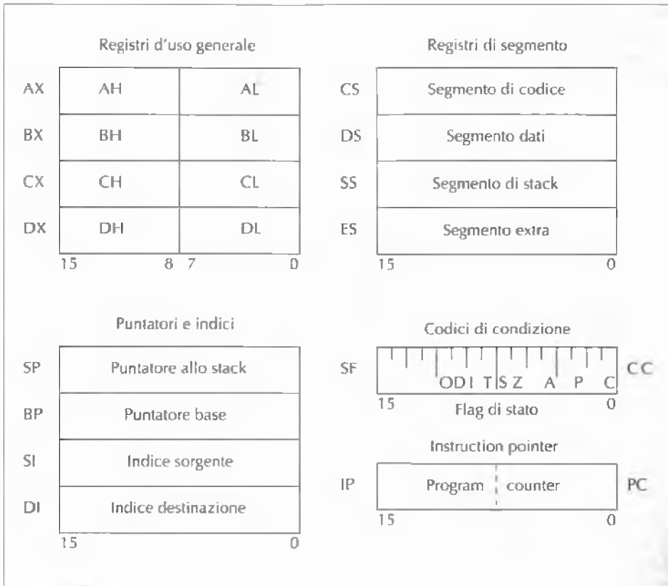
Figura C.2 Registri dell'8088.
