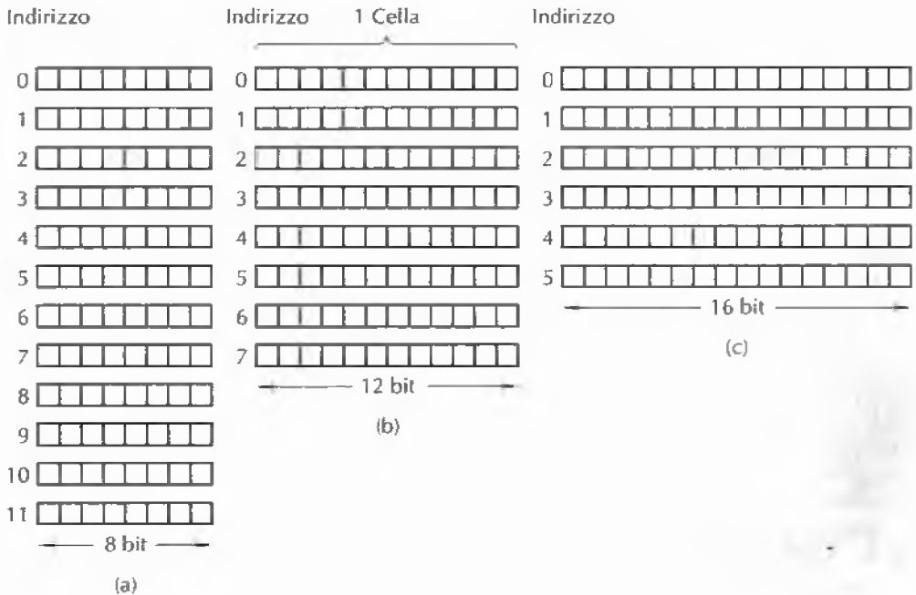
Figura 2.9 Tre modi di organizzare una memoria a 96 bit.
