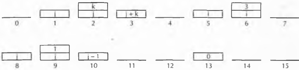
Figura 4.15 Stack dopo ogni istruzione della Figura 4.14(b).
