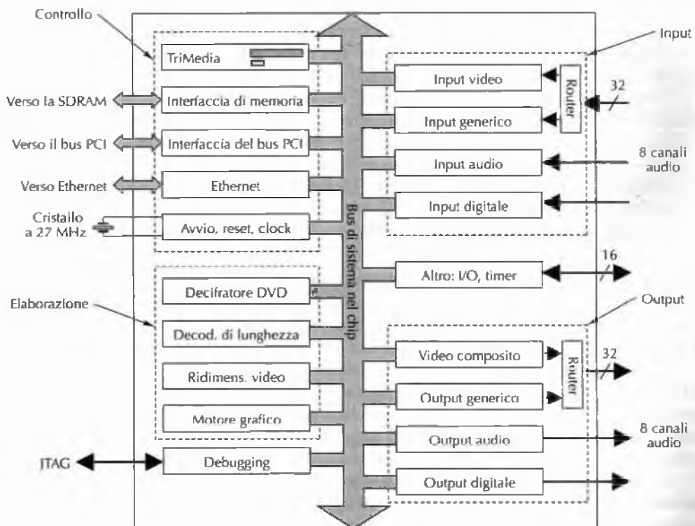
Figura 8.16 Multiprocessore eterogeneo nel chip Nexperia.
