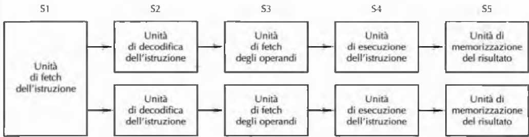
Figura 2.5 Doppia pipeline a cinque stadi con l'unità di fetch dell'istruzione in comune.
