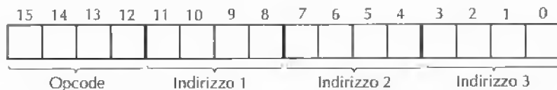
Figura 5.12 Un'istruzione composta da un opcode di 4 bit e da tre campi d'indirizzo di 4 bit.
