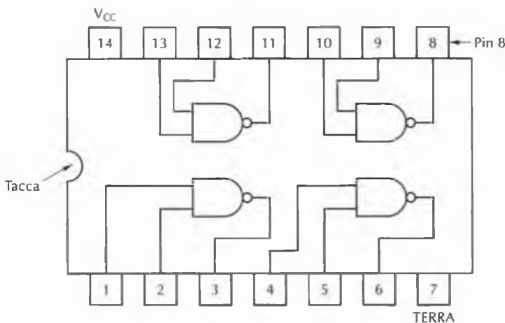
Figura 3.10 Chip SSI con quattro porte logiche.
