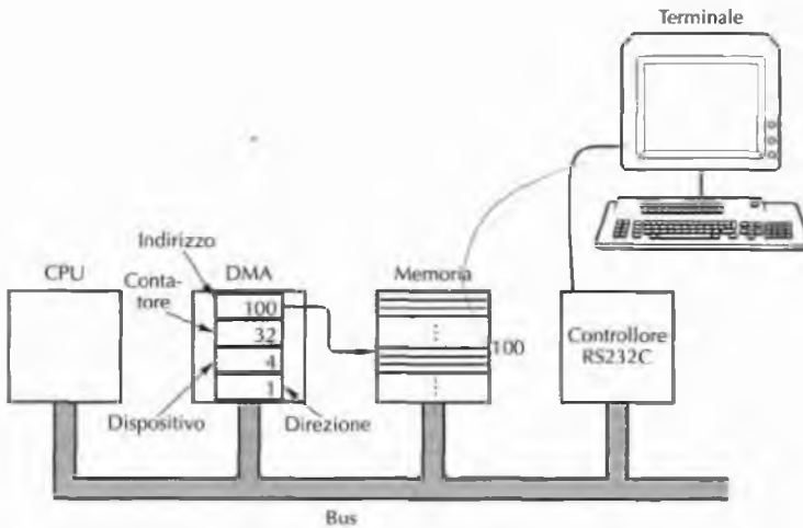
Figura 5.33 Controllore DMA.
