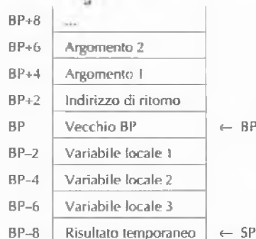
Figura C.6 Un esempio di stack durante l'esecuzione di una subroutine.
