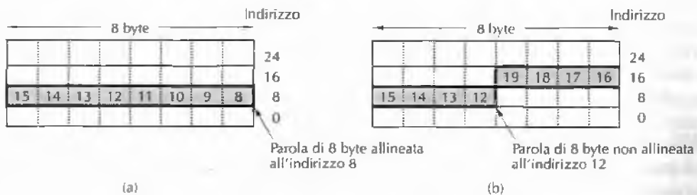
Figura 5.2 Una parola di 8 byte in una memoria little-endian (a) allineata e (b) non allineata. Alcune macchine richiedono che le parole siano allineate.
