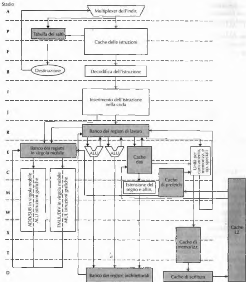
Figura 4.49 Rappresentazione semplificata della pipeline dell'UltraSPARC III Cu.
