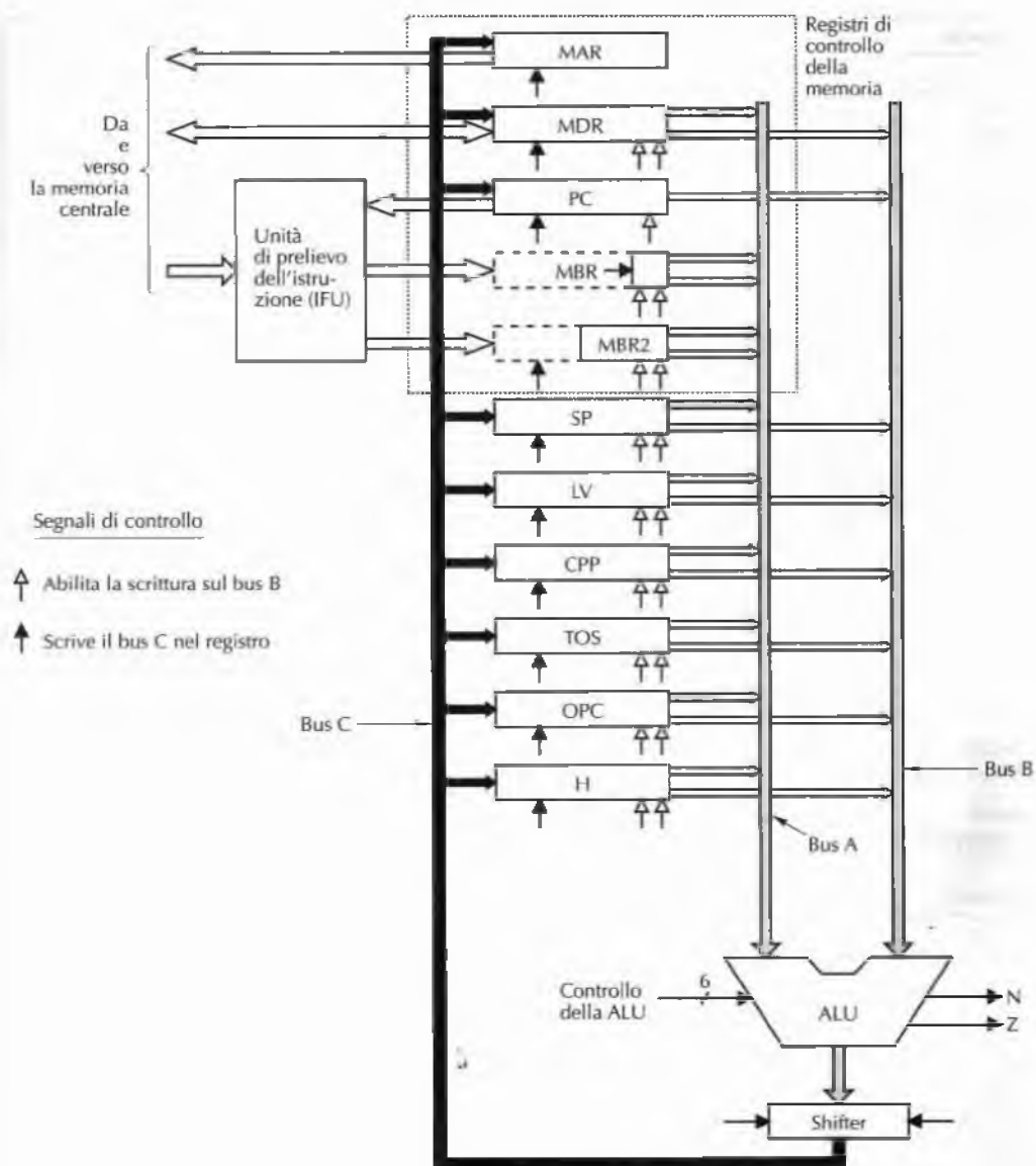
Figura 4.29 Percorso dati di Mic-2.
