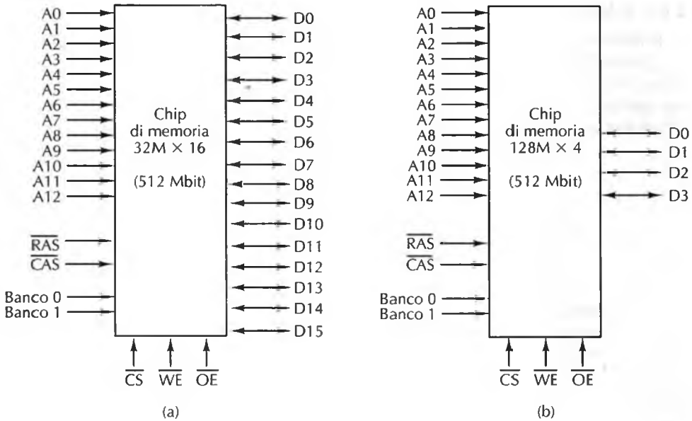
Figura 3.32 Due modi di organizzare un chip di memoria a 512 Mbit.
