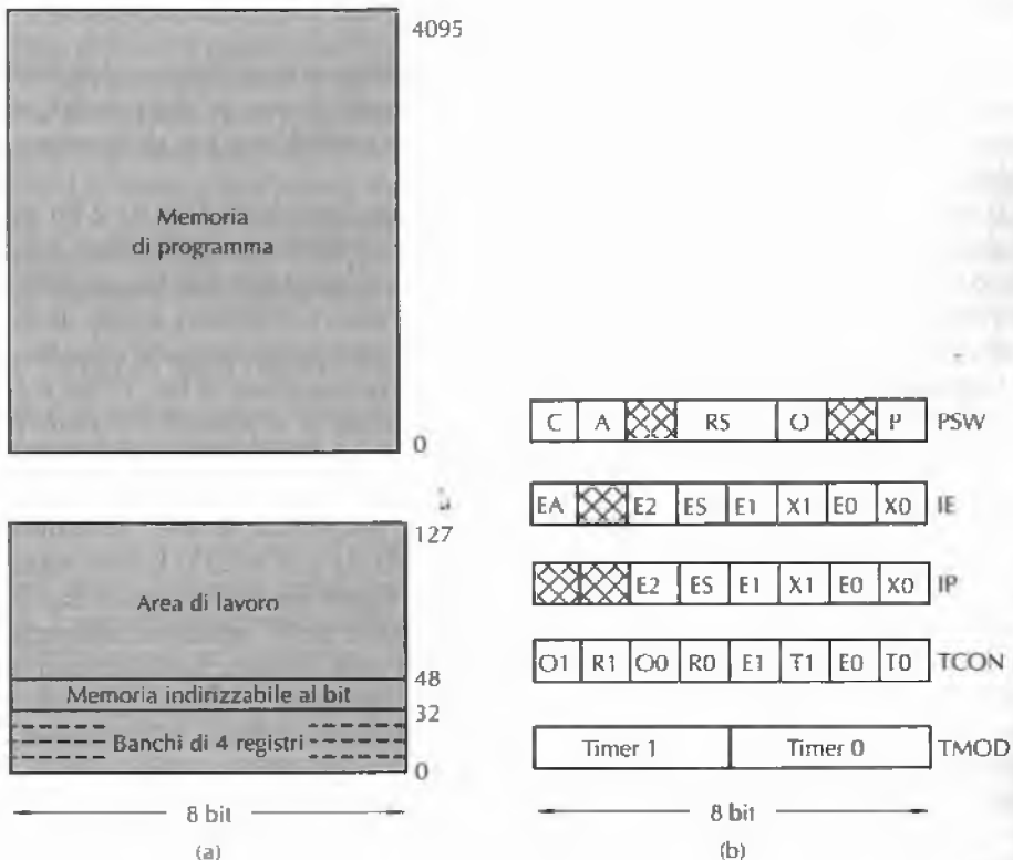
Figura 5.6 (a) Organizzazione della memoria su chip dell'8051. (b) Registri principali dell'8051.
