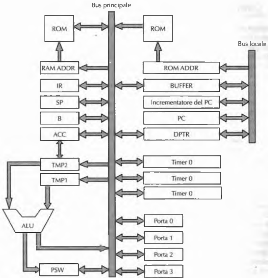
Figura 4.50 Microarchitettura dell'8051.
