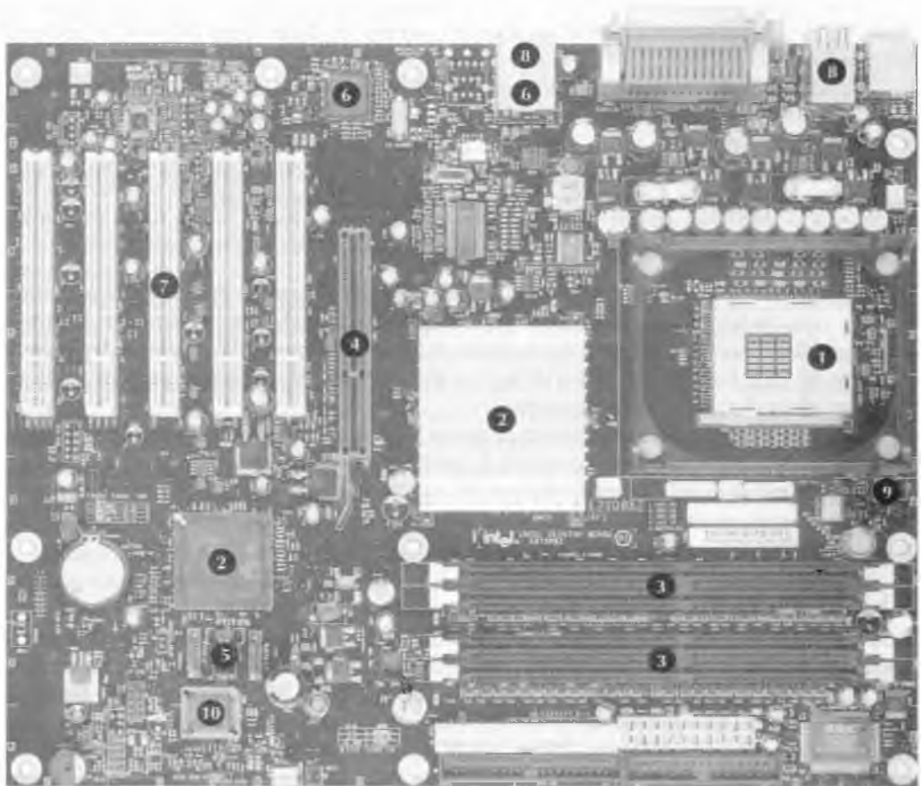
Figura 1.10 Nel cuore di ogni personal computer c'è una scheda di circuiti stampati. Questa immagine è una fotografia della scheda Intel D875PBZ. La fotografia è di proprietà di Intel Corporation (copyright 2003) e pubblicata con autorizzazione.
