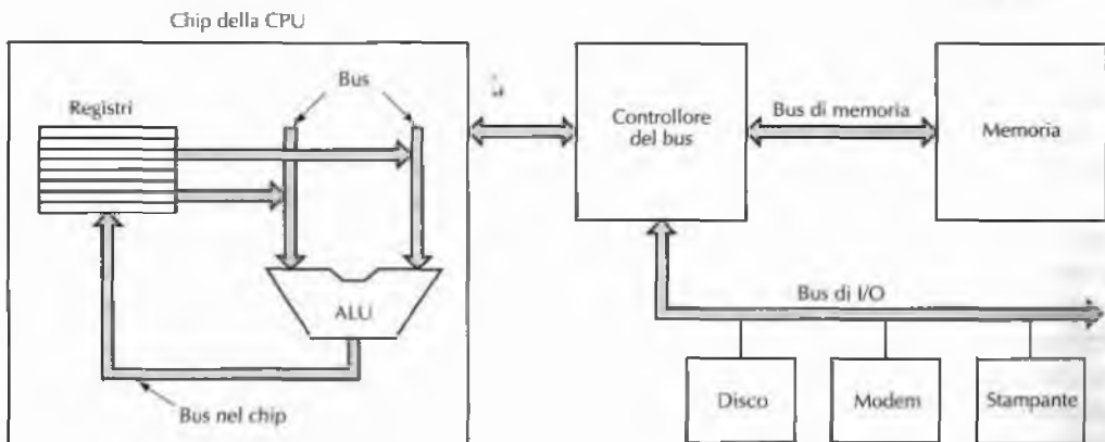
Figura 3.35 Sistema di un calcolatore con più bus.
