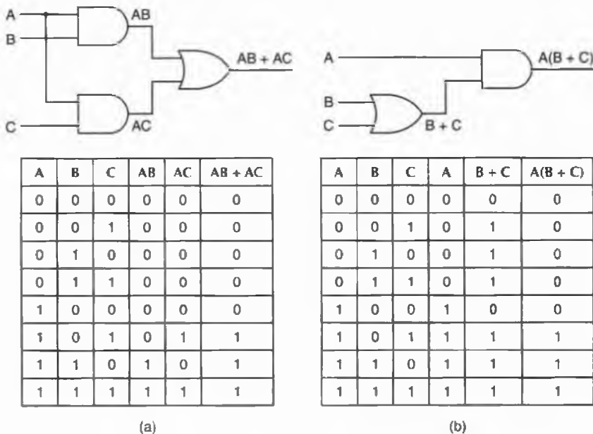
Figura 3.5 Due funzioni equivalenti. (a) AB + AC . (b) A(B + C) .
