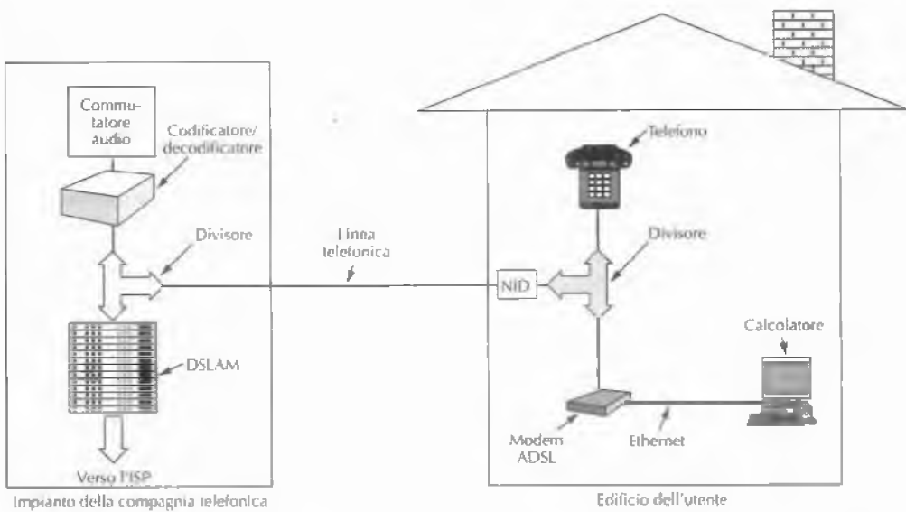
Figura 2.39 Tipica configurazione dei dispositivi per la ADSL.
