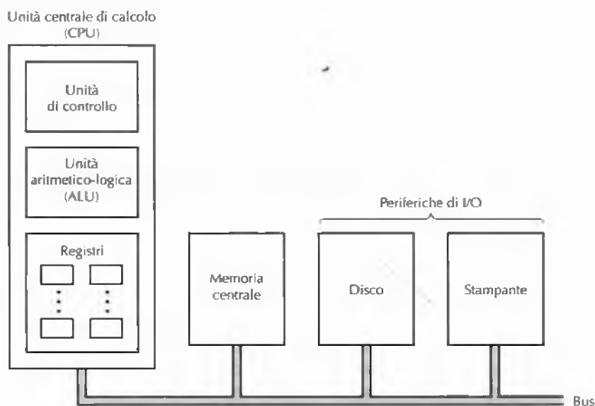
Figura 2.1 Organizzazione di un semplice calcolatore con una CPU e due periferiche di I/O.
