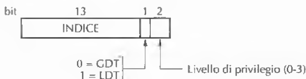
Figura 6.12 Selettore del Pentium 4.
