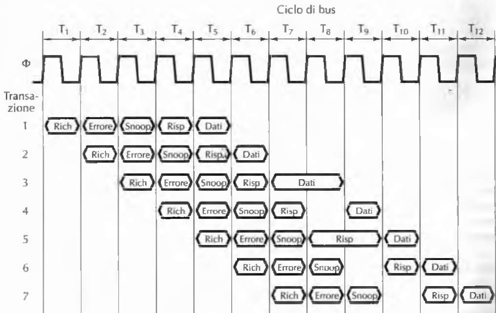
Figura 3.46 Richieste organizzate a pipeline sul bus di memoria del Pentium 4.
