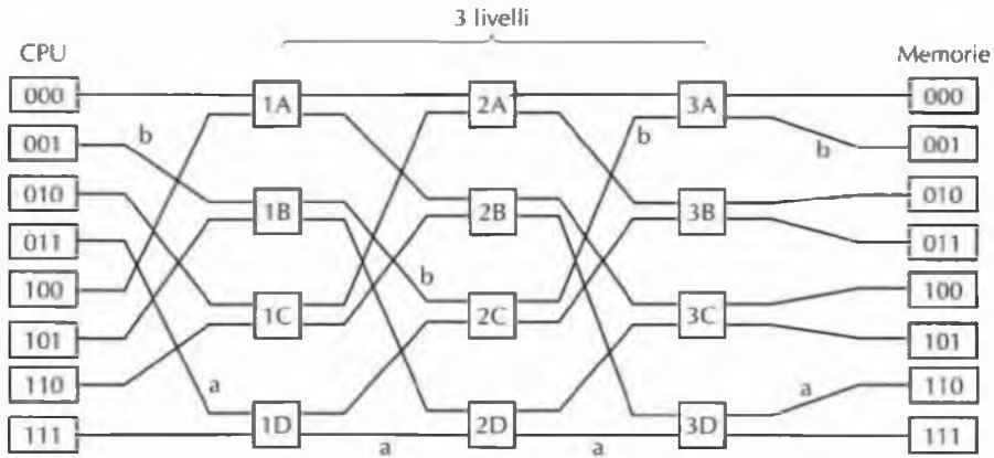
Figura 8.29 Rete di connessione omega.
