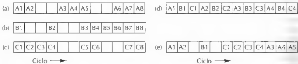
Figura 8.7 (a)-(c) Tre thread: le caselle vuote indicano che il thread è in stallo perché in attesa di dati dalla memoria. (d) Multithreading a grana fine. (e) Multithreading a grana grossa.
