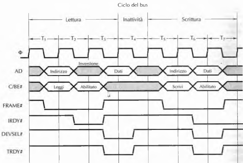
Figura 3.56 Esempi di transazioni di un bus PCI a 32 bit. I primi tre cicli sono utilizzati per un'operazione di lettura. Segue un ciclo d'inattività e infine tre cicli per un'operazione di scrittura.
