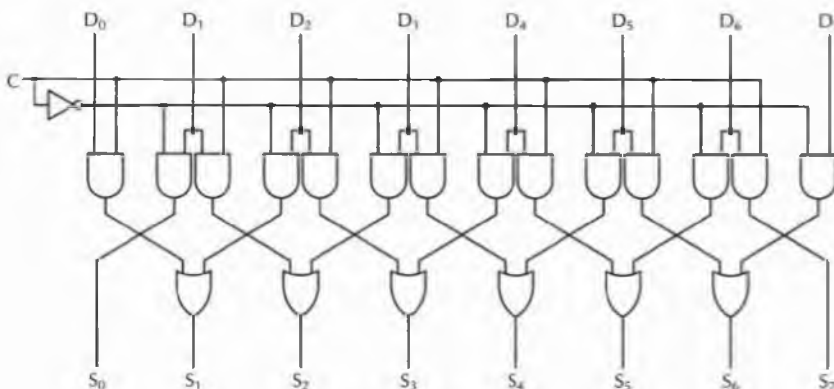
Figura 3.16 Registro a scorrimento a sinistra di 1 bit.
