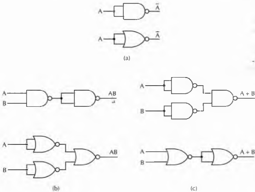
Figura 3.4 Costruzione delle porte logiche (a) NOT, (b) AND e (c) OR utilizzando soltanto porte NOR.
