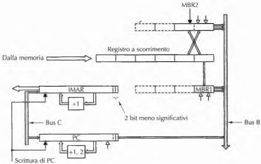
Figura 4.27 Unità di prelievo per Mic-1.
