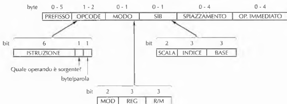
Figura 5.14 Formati d'istruzione di Pentium 4.
