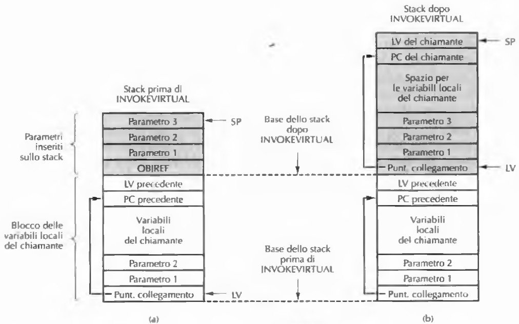
Figura 4.12 (a) Memoria prima di eseguire l'istruzione INVOKEVIRTUAL . (b) Dopo averla eseguita.
