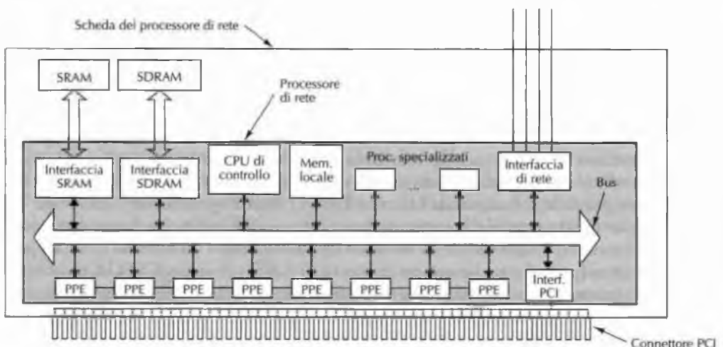
Figura 8.15 Scheda e chip di un comune processore di rete.
