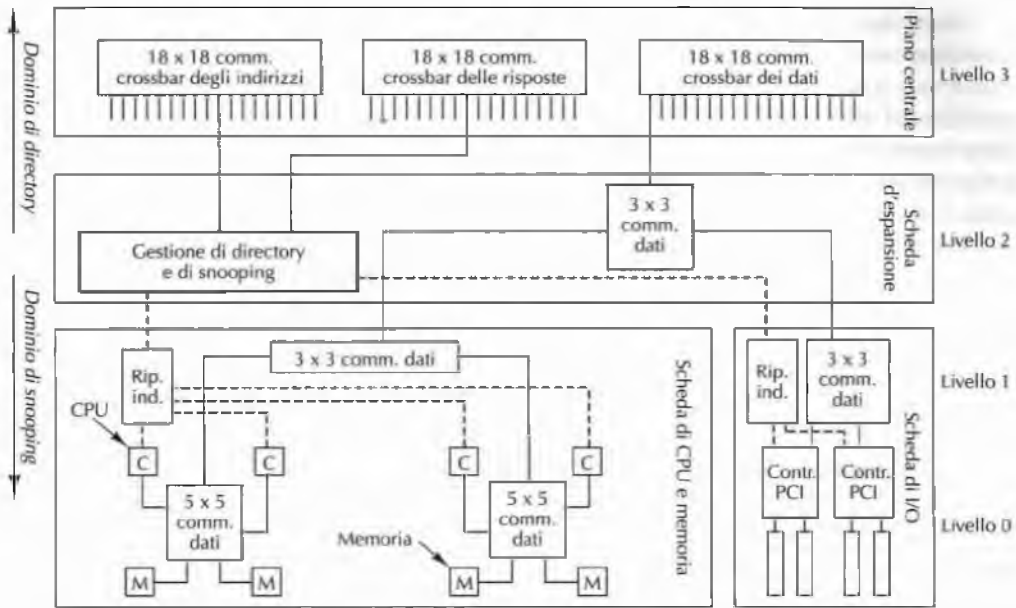
Figura 8.33 Sun Fire E25K usa un'interconnessione a quattro livelli. Le linee tratteggiate rappresentano i percorsi degli indirizzi, quelle continue i percorsi dei dati.
