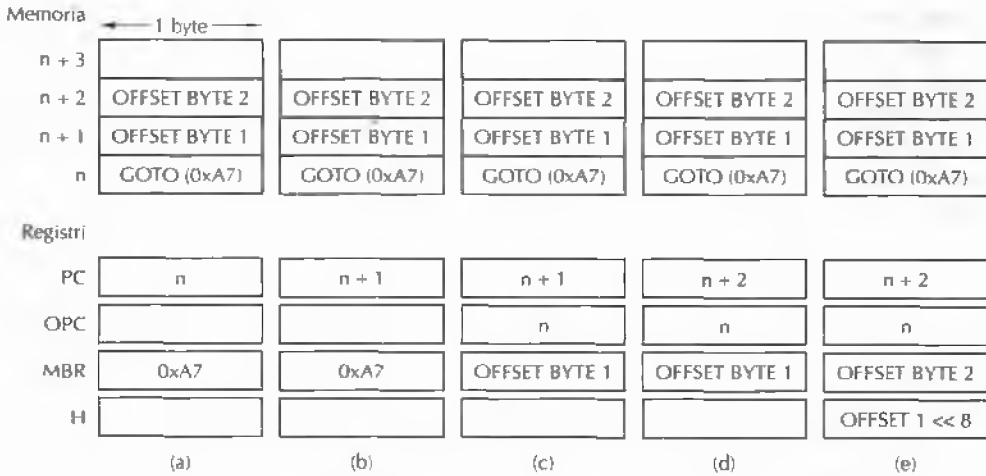
Figura 4.22 Situazione all'inizio di alcune microistruzioni. (a) main1 . (b) goto1 . (c) goto2 . (d) goto3 . (e) goto4 .
