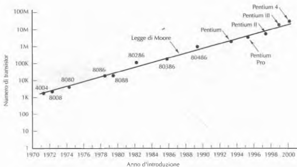
Figura 1.13 La legge di Moore per i chip della CPU (Intel).
