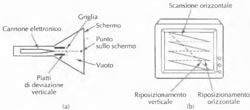
Figura 2.31 (a) Spaccato di un CRT. (b) Scansione di un CRT.
