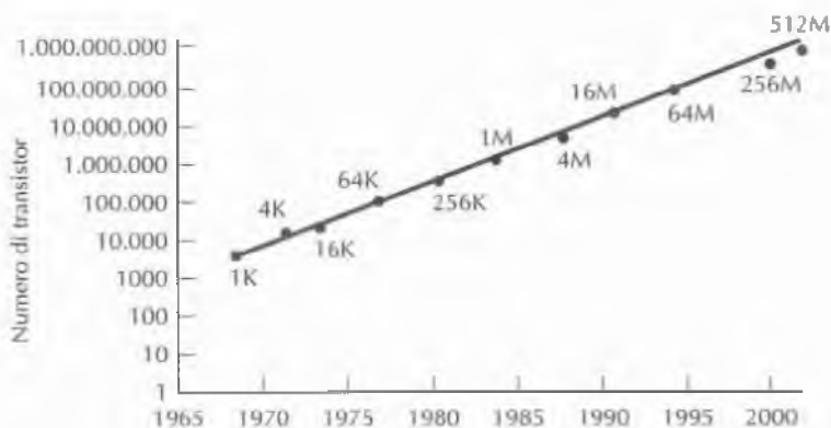
Figura 1.8 La legge di Moore prevede un aumento annuale del 60% del numero di transistor che può essere inserito su un chip. I valori presenti vicino ai punti del grafico rappresentano le dimensioni della memoria, in bit.
