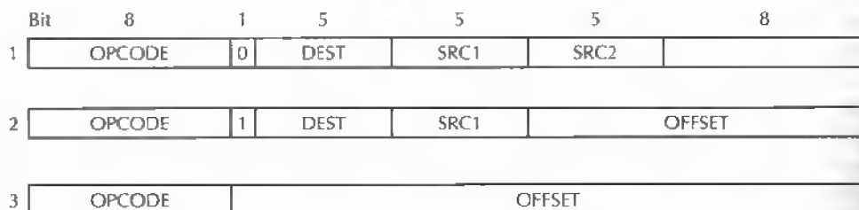
Figura 5.25 Semplice progetto dei formati d'istruzione di una macchina a tre indirizzi.
