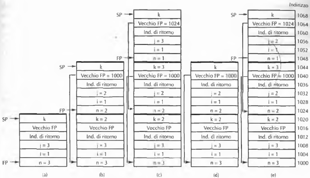
Figura 5.43 Lo stack in alcuni momenti dell'esecuzione del codice della Figura 5.42.
