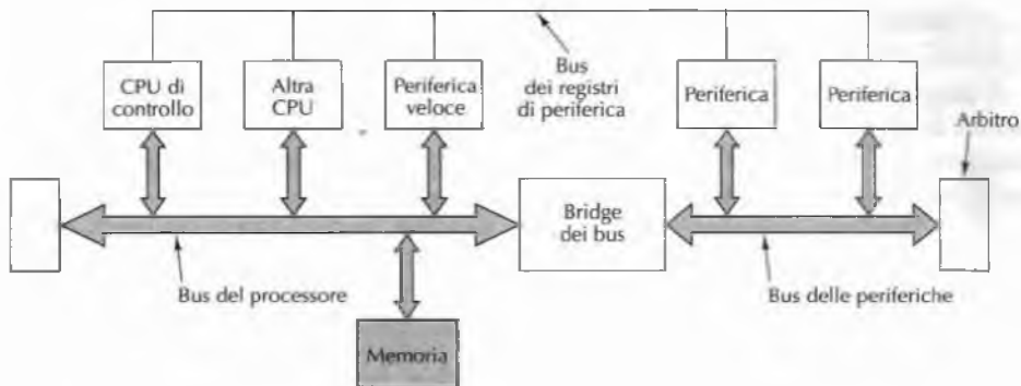
Figura 8.12 Esempio di architettura CoreConnect di IBM.
