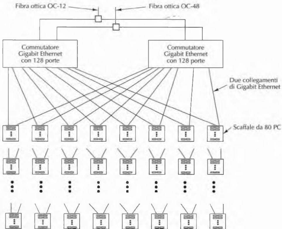
Figura 8.42 Un tipico cluster di Google.
