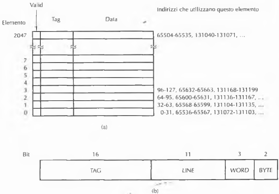
Figura 4.38 (a) Cache a corrispondenza diretta. (b) Indirizzo virtuale a 32 bit.
