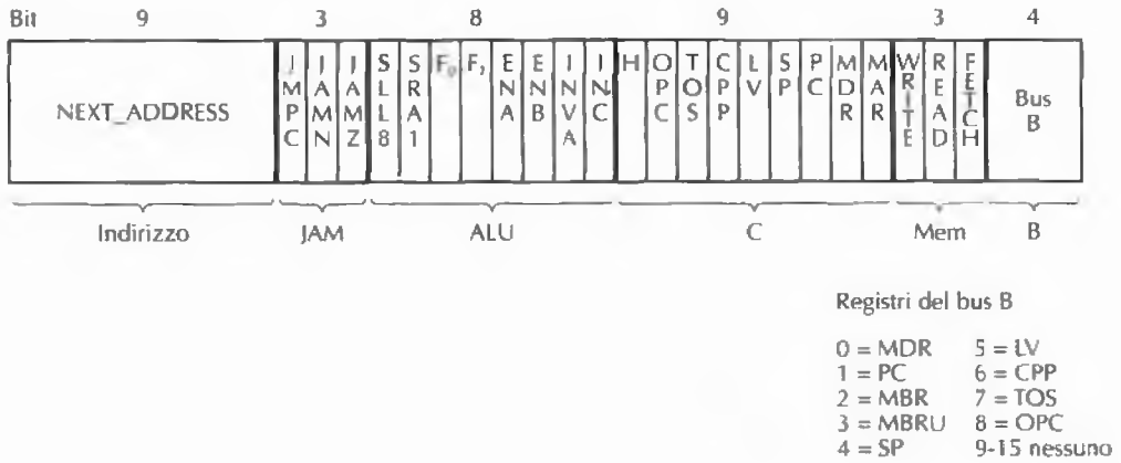
Figura 4.5 Formato delle microistruzioni di Mic-1.
