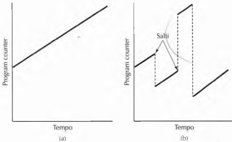
Figura 5.39 Valore del program counter in funzione del tempo. (a) Senza salti. (b) Con salti.
