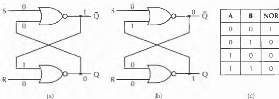
Figura 3.22 (a) Latch di tipo NOR nello stato 0. (b) Latch di tipo NOR nello stato 1. (c) Tabella di verità del NOR.
