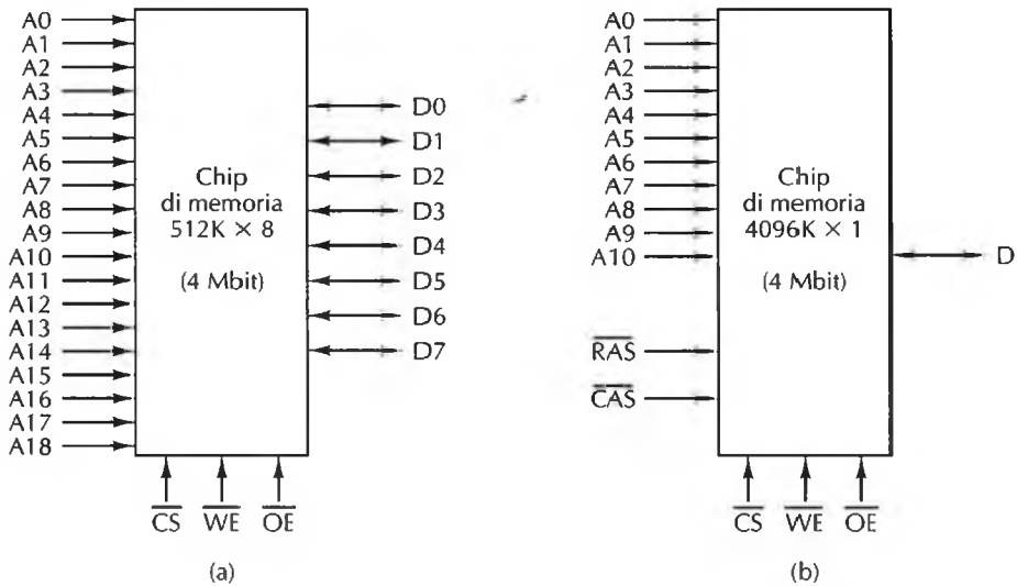
Figura 3.31 Due modi di organizzare un chip di memoria a 4 Mbit.
