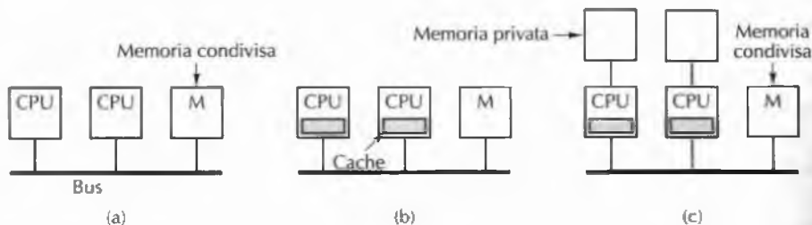
Figura 8.24 Tre multiprocessori basati su bus. (a) Senza caching. (b) Con caching. (c) Con caching e memorie private.
