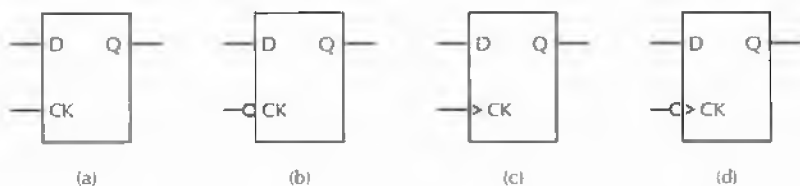
Figura 3.27 Flip-flop D temporizzati.
