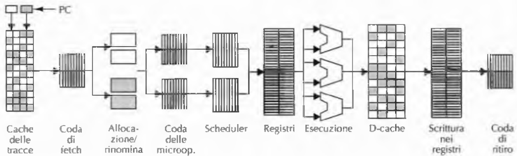
Figura 8.9 Condivisione delle risorse tra i thread della microarchitettura Netburst del Pentium 4.
