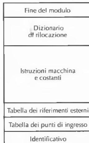
Figura 7.16 Struttura interna di un modulo oggetto prodotto da un traduttore.
