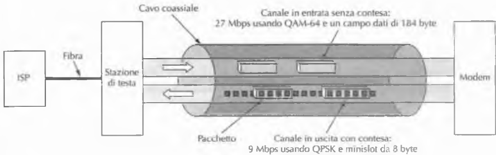
Figura 2.41 Tipici dettagli dei canali in entrata e in uscita nel Nord America.
