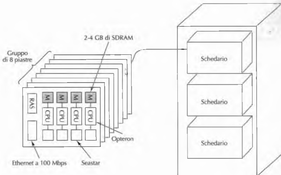
Figura 8.38 Assemblaggio dei componenti di un Red Storm.
