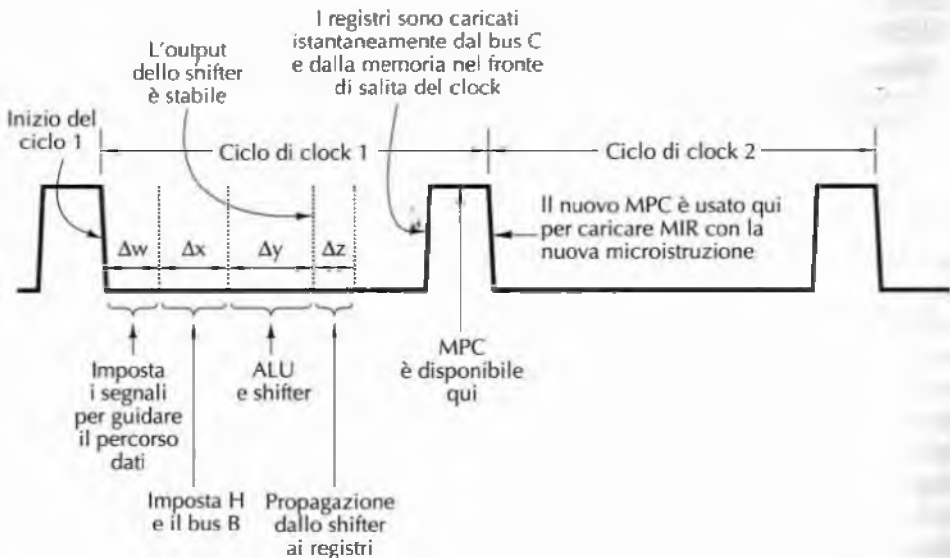
Figura 4.3 Temporizzazione di un ciclo di clock del percorso dati.
