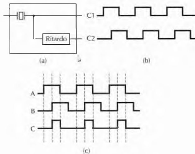
Figura 3.21 (a) Clock. (b) Diagramma di temporizzazione del clock. (c) Generazione di un clock asimmetrico.
