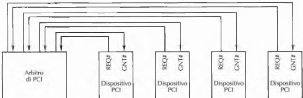
Figura 3.54 Il bus PCI utilizza un arbitro del bus centralizzato.
