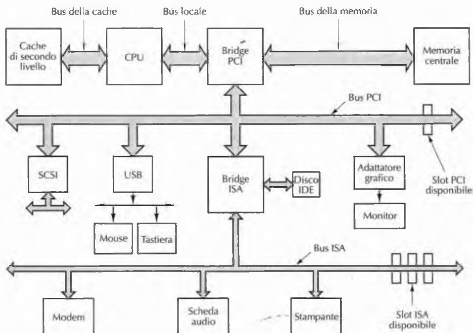
Figura 3.52 Architettura di uno dei primi Pentium. I bus più spessi hanno una maggiore larghezza di banda rispetto a quelli più sottili (la figura non è in scala).
