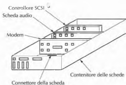
Figura 2.28 Struttura fisica di un personal computer.
