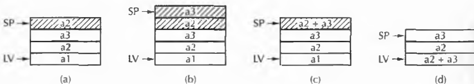
Figura 4.9 Utilizzo dello stack degli operandi per il calcolo di un'espressione aritmetica.
