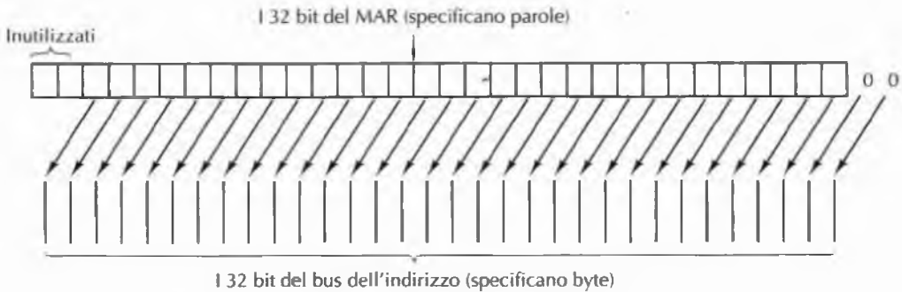
Figura 4.4 Corrispondenza tra i bit di MAR e i bit del bus dell'indirizzo.
