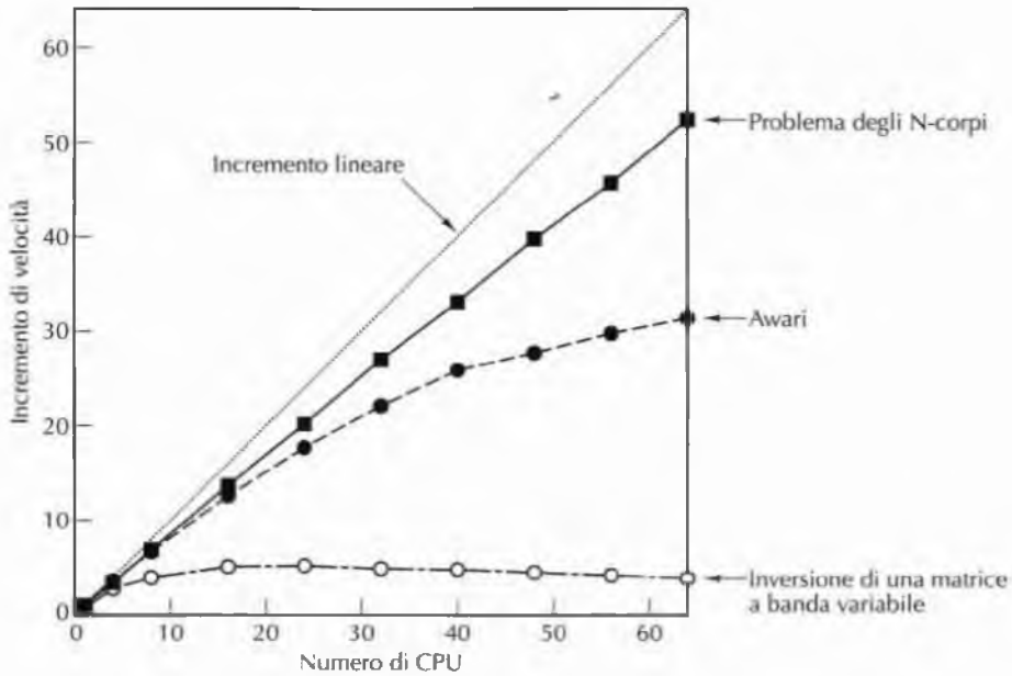
Figura 8.47 I programmi reali hanno incrementi di velocità minori di quello ideale (linea punteggiata).
