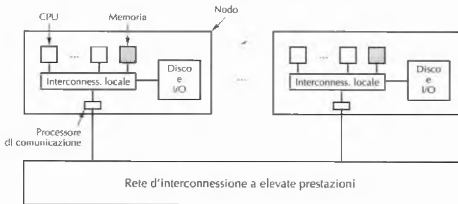
Figura 8.34 Schema di un multicomputer.
