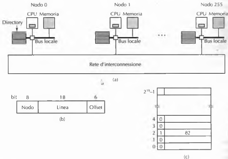
Figura 8.31 (a) Multiprocessore di 256 nodi basato su directory. (b) Divisione in campi di un indirizzo di memoria di 32 bit. (c) Directory in corrispondenza del nodo 36.
