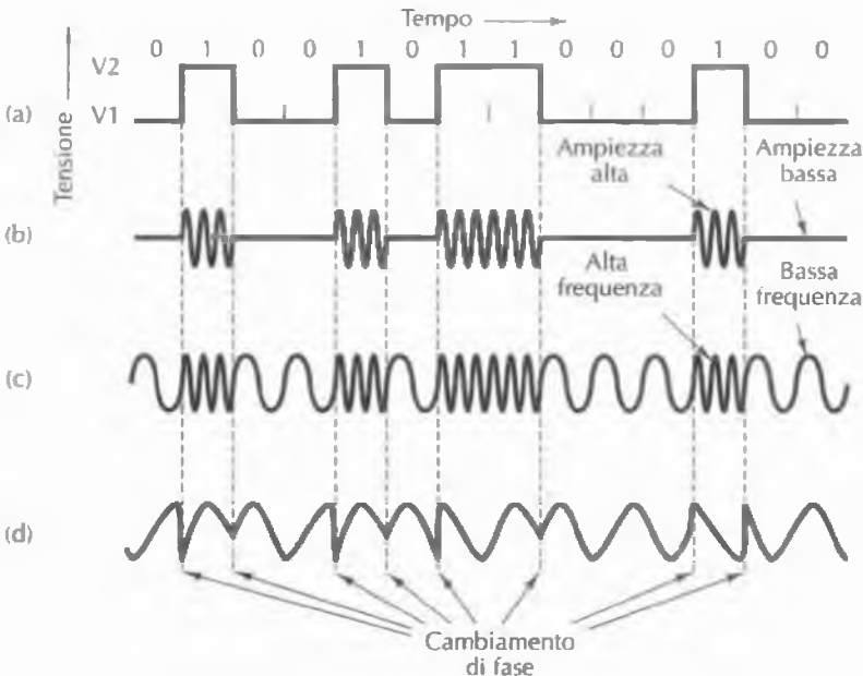
Figura 2.37 Trasmissione bit a bit della stringa 01001011000100 su una linea telefonica. (a) Segnale a due livelli. (b) Modulazione d'ampiezza. (c) Modulazione di frequenza. (d) Modulazione di fase.
