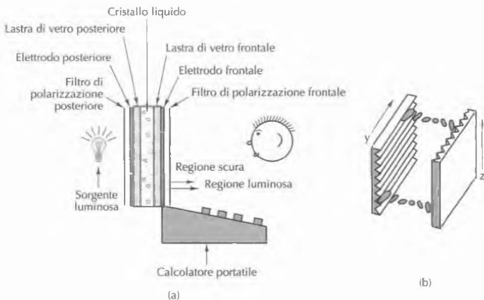
Figura 2.32 (a) Struttura di uno schermo LCD. (b) I solchi sulla lastra frontale e su quella posteriore sono perpendicolari tra loro.
