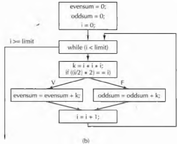
Figura 4.45 (a) Frammento di programma. (b) Grafico a blocchi corrispondente.
