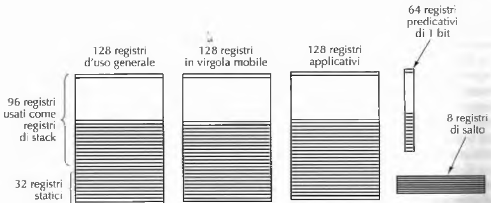
Figura 5.49 Registri di Itanium 2.
