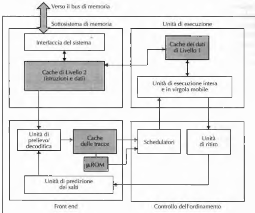
Figura 4.46 Diagramma a blocchi del Pentium 4.
