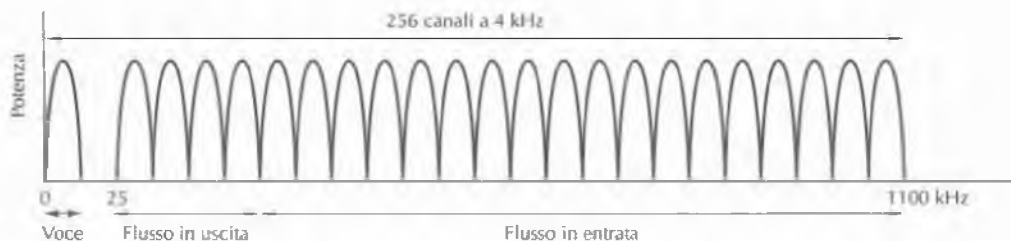
Figura 2.38 Funzionamento di una ADSL.
