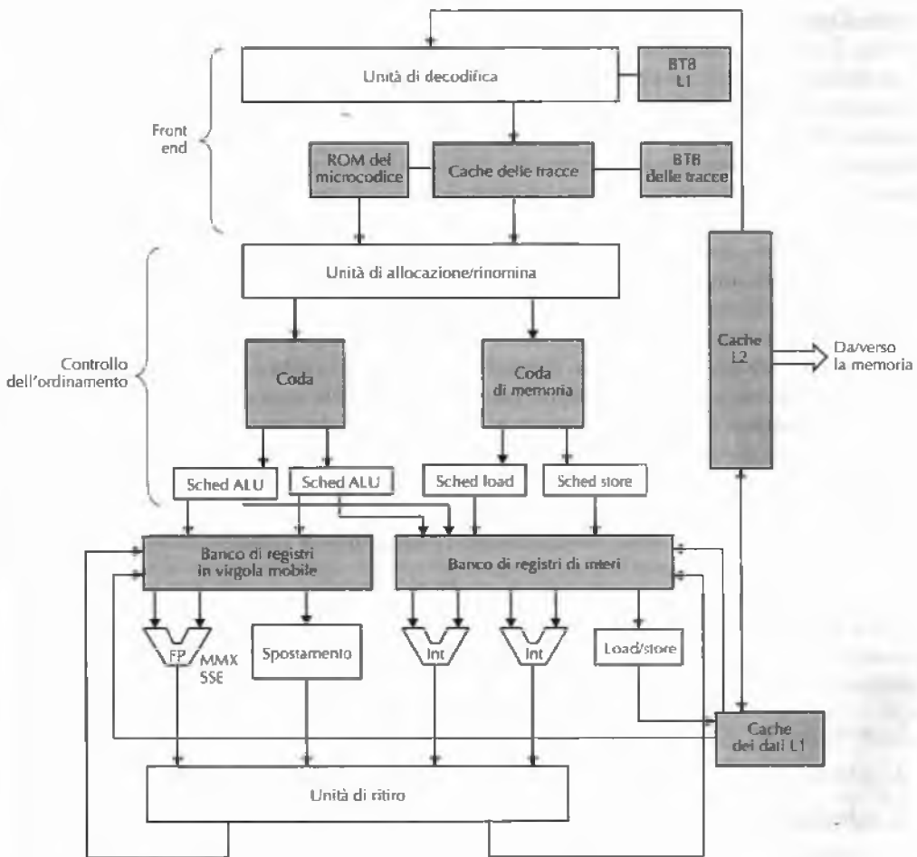
Figura 4.47 Vista semplificata del percorso dati del Pentium 4.
