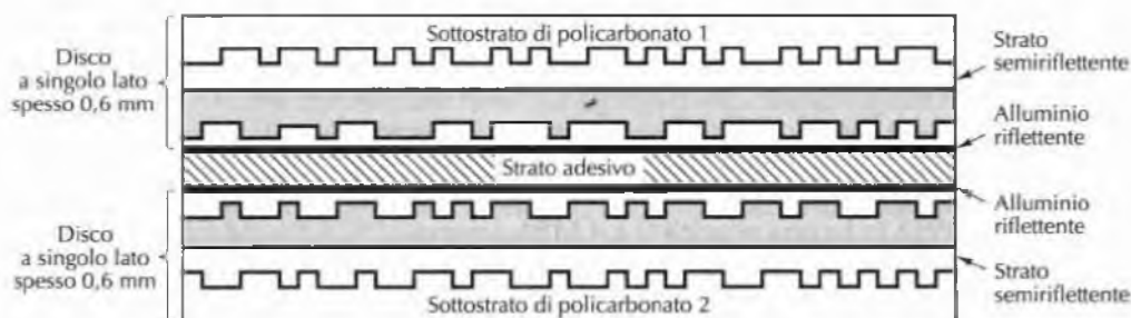
Figura 2.27 Disco DVD a doppio lato e doppio strato.
