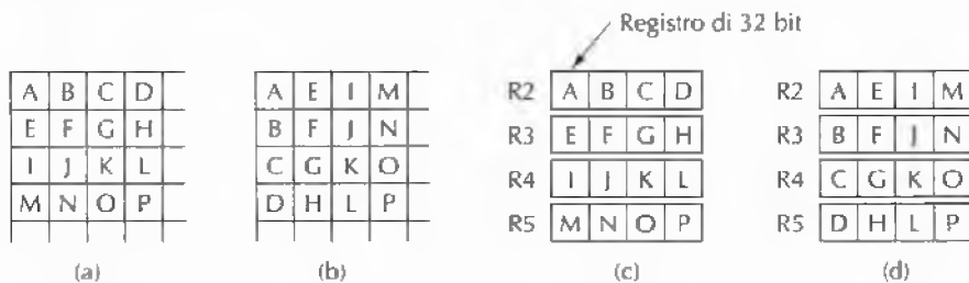
Figura 8.6 (a) Un array di elementi di 8 bit. (b) L'array trasposto. (c) L'array originale memorizzato in quattro registri. (d) L'array trasposto nei quattro registri.
