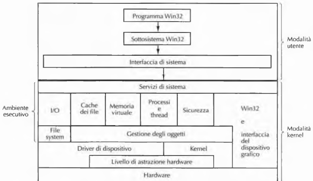
Figura 6.31 Struttura di Windows XP.
