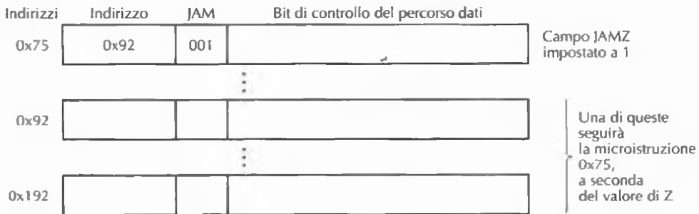
Figura 4.7 Le microistruzioni con JAMZ = 1 hanno due possibili successori.
