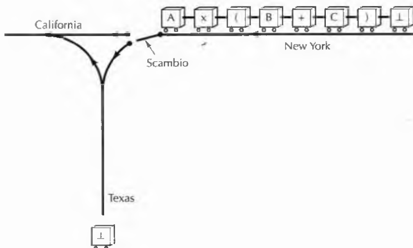
Figura 5.21 Ogni vagone ferroviario rappresenta un simbolo della formula infissa da convertire in notazione polacca inversa.
