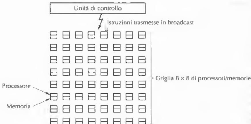
Figura 2.7 Array di processori del tipo ILLIAC IV.
