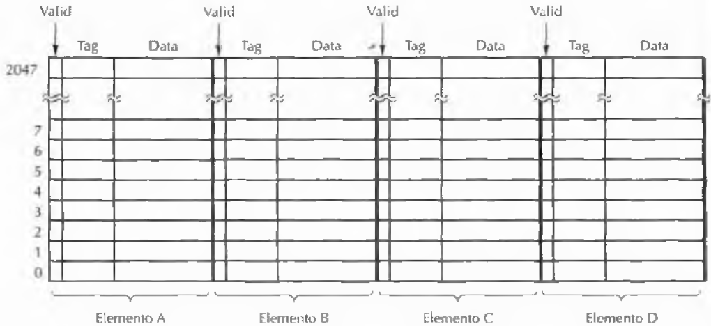
Figura 4.39 Cache associativa a quattro vie.
