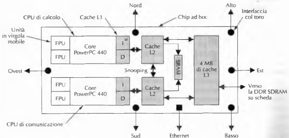
Figura 8.36 Il chip costruito per BlueGene/L.
