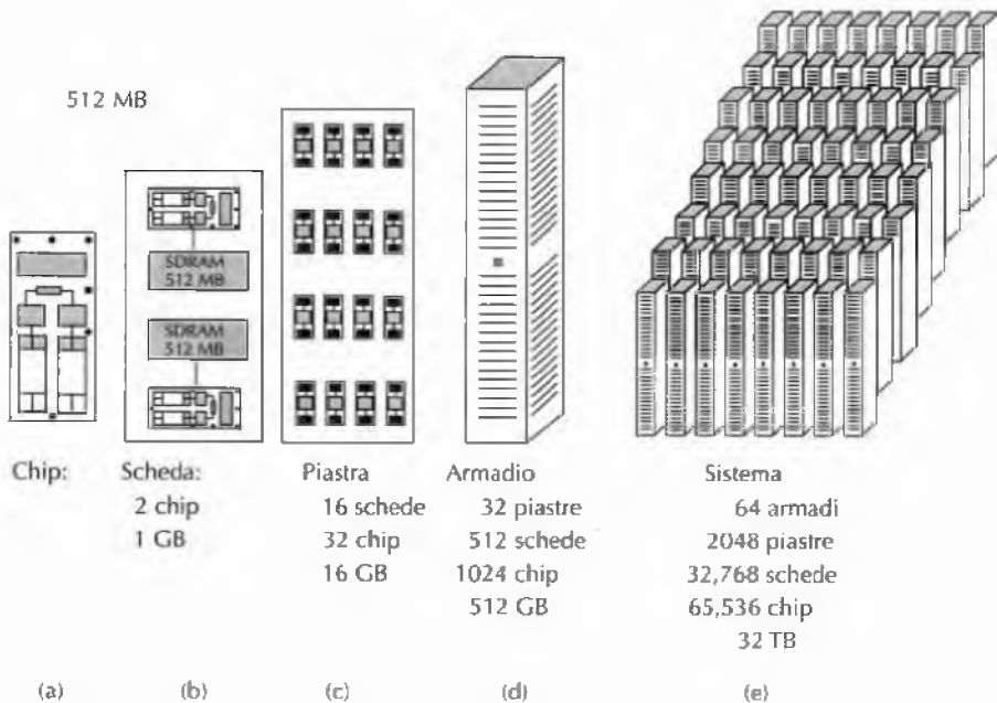
Figura 8.37 Componenti gerarchiche di BlueGene/L: (a) Chip (b) Scheda (c) Piastra (d) Armadio (e) Sistema.
