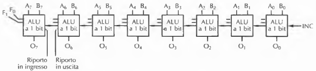
Figura 3.20 Otto ALU a 1 bit connesse per comporre una ALU a 8 bit. Per semplificare non sono mostrati segnali di abilitazione e segnali di inversione.
