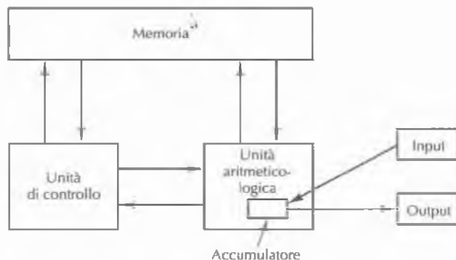
Figura 1.5 La macchina originale di von Neumann.
