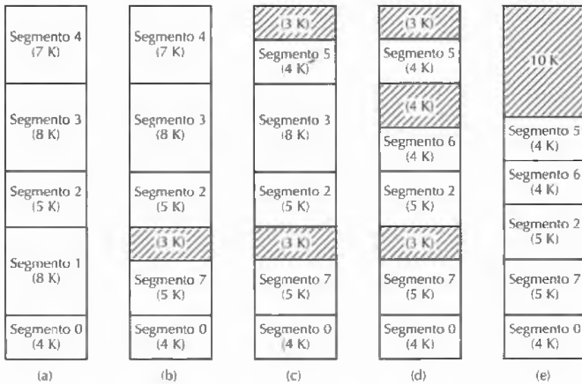
Figura 6.10 (a)-(d) Incremento della frammentazione esterna. (e) Rimozione della frammentazione esterna mediante compattamento.
