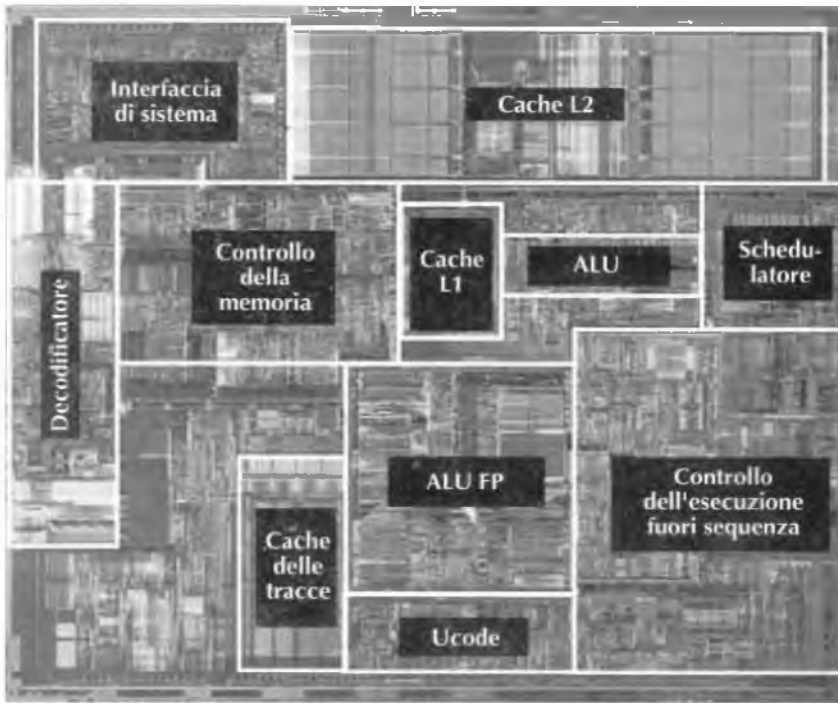
Figura 1.12 Il chip Pentium 4. La fotografia è di proprietà di Intel Corporation (copyright 2003) e pubblicata con autorizzazione.
