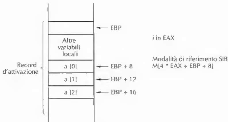
Figura 5.28 Accesso ad a[i] .
