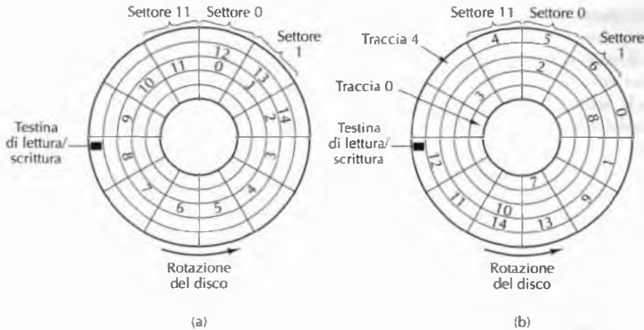
Figura 6.20 Strategie di allocazione su disco. (a) Un file in settori consecutivi. (b) Un file in settori non consecutivi.
