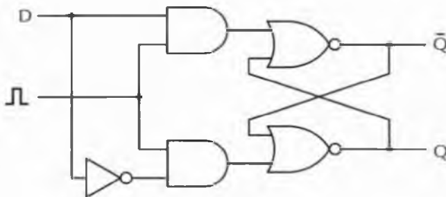
Figura 3.24 Latch D temporizzato.
