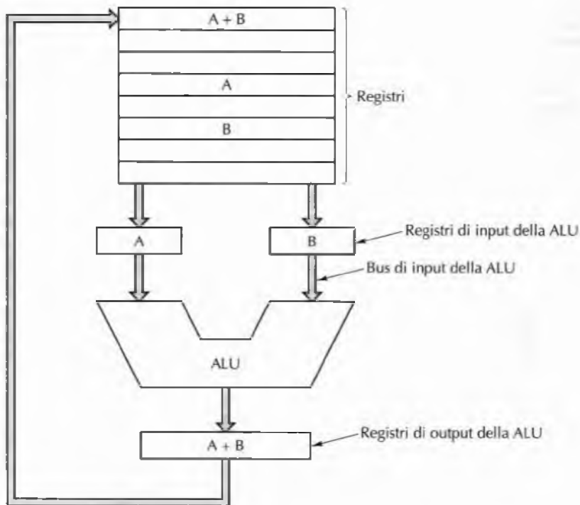
Figura 2.2 Percorso dati di una tipica macchina di von Neumann.
