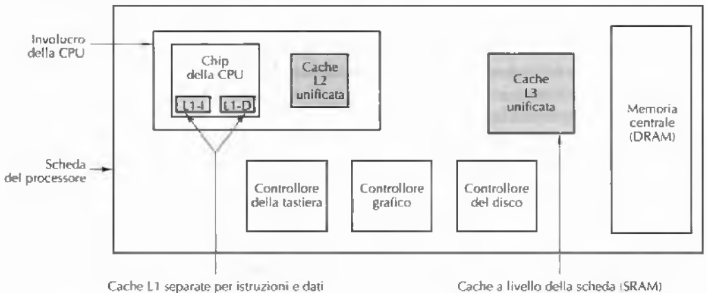
Figura 4.37 Sistema con tre livelli di cache.
