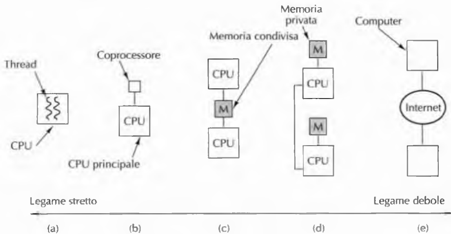
Figura 8.1 (a) Parallelismo nel chip. (b) Coprocessore. (c) Multiprocessore. (d) Multicomputer. (e) Griglia.
