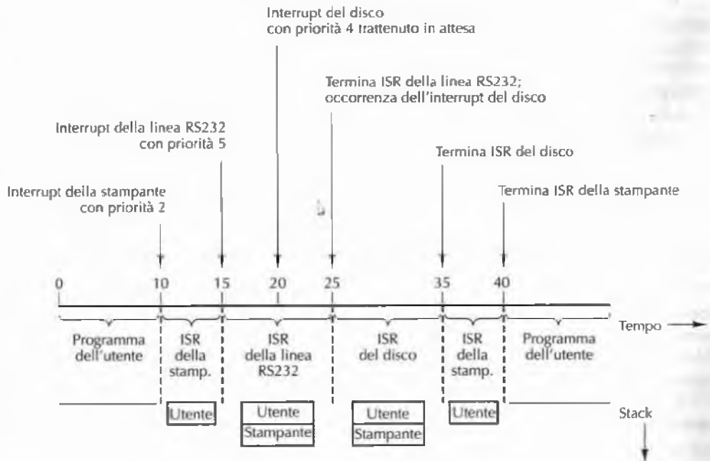
Figura 5.46 Sequenza di interrupt.
