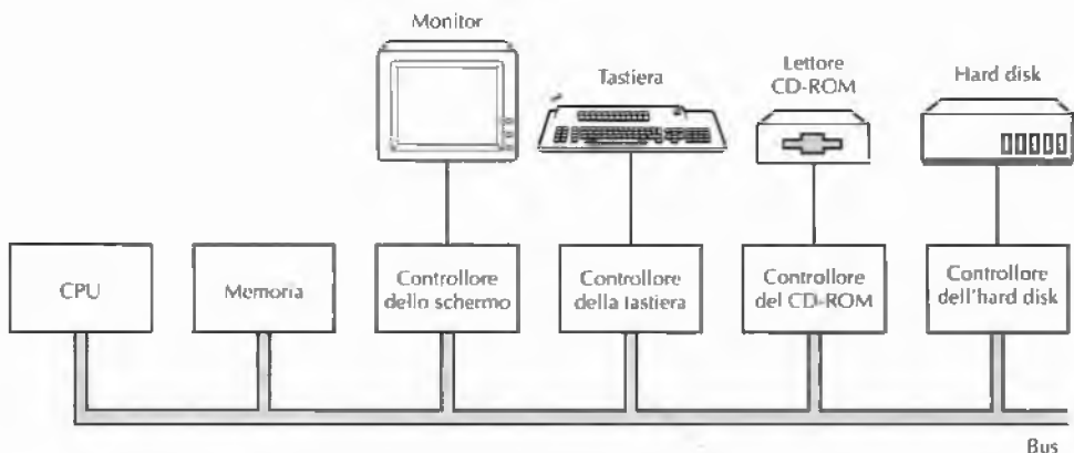
Figura 2.29 Struttura logica di un semplice personal computer.
