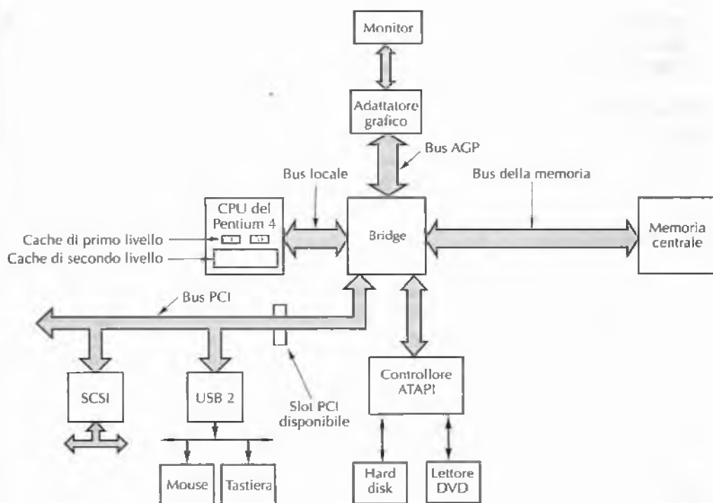
Figura 3.53 Struttura del bus di un moderno Pentium 4.
