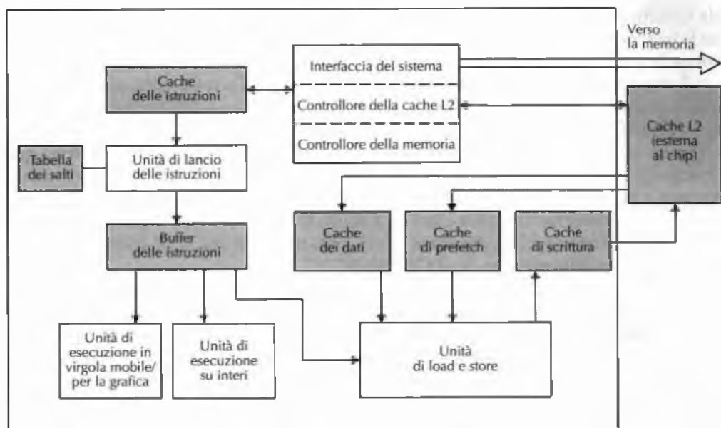
Figura 4.48 Diagramma a blocchi dell'UltraSPARC III Cu.
