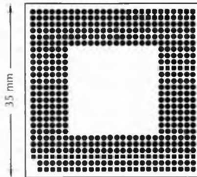
Figura 3.44 Disposizione fisica dei contatti del Pentium 4.
