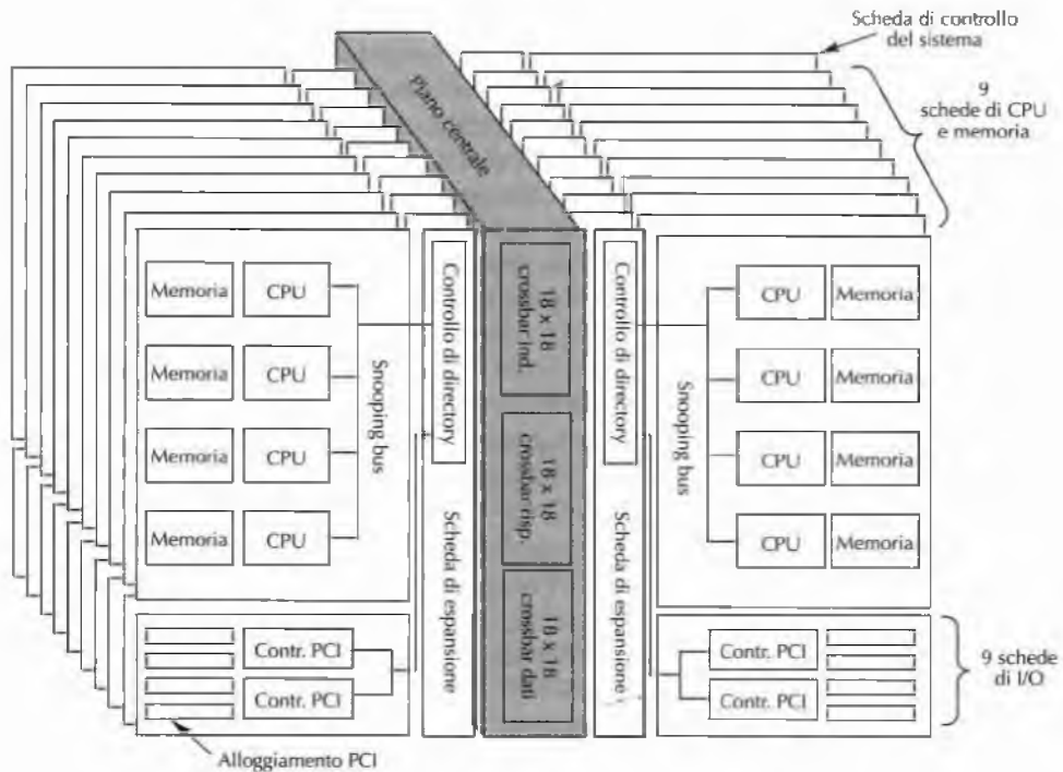
Figura 8.32 Multiprocessore E25K di Sun Microsystems.
