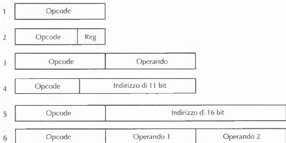
Figura 5.16 Formati d'istruzione di 8051.
