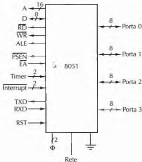
Figura 3.50 Disposizione logica dei contatti dell'8051.
