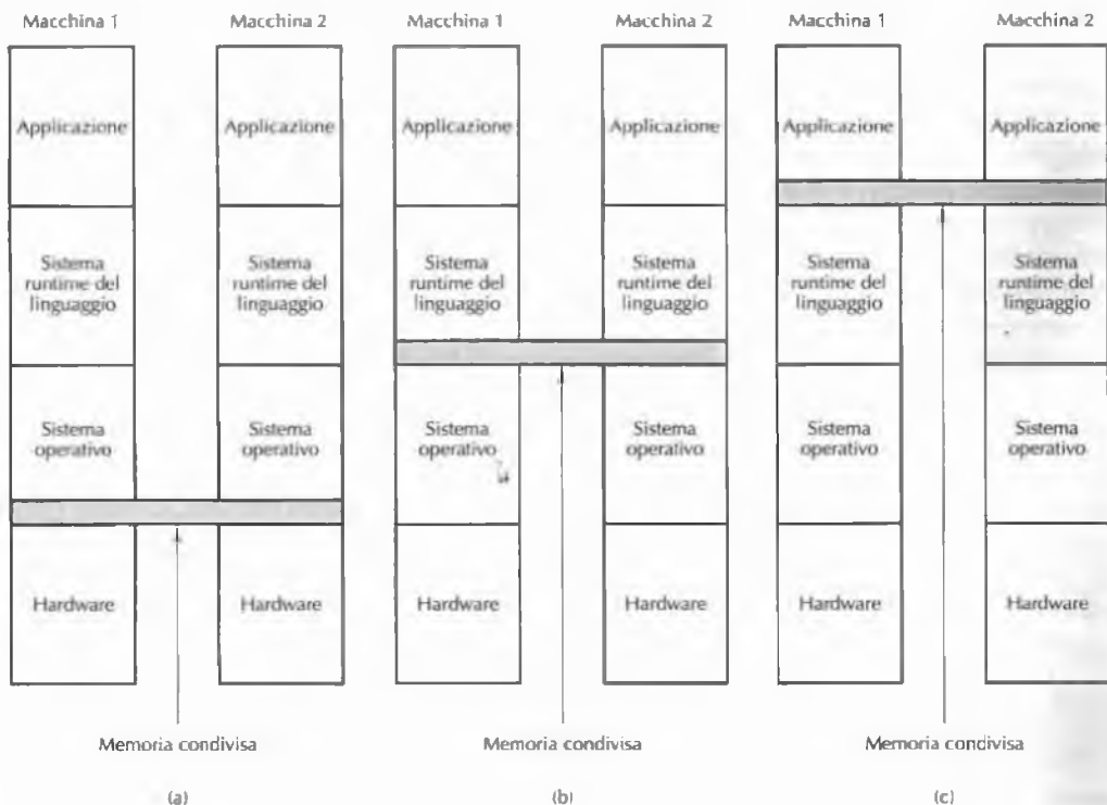
Figura 8.19 Vari livelli d'implementazione di una memoria condivisa. (a) Nell'hardware. (b) Nel sistema operativo. (c) Nel sistema runtime del linguaggio.
