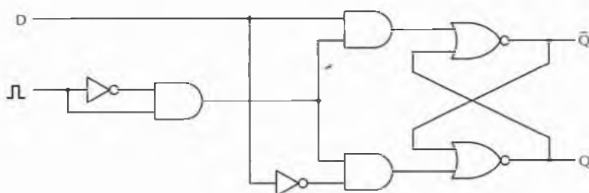
Figura 3.26 Flip-flop D.
