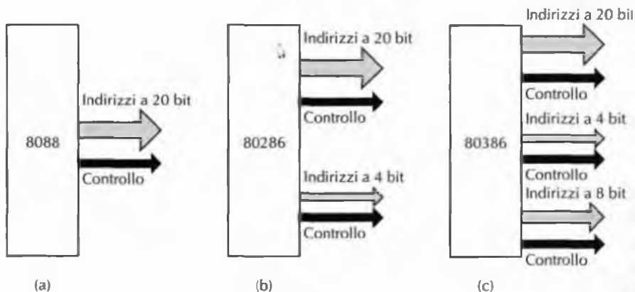
Figura 3.37 Crescita nel tempo degli indirizzi del bus.
