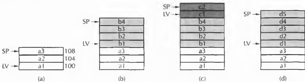
Figura 4.8 Utilizzo dello stack per memorizzare le variabili locali. (a) Mentre A è attiva. (b) Dopo che A ha richiamato B . (c) Dopo che B ha richiamato C . (d) Dopo che C e B hanno restituito il controllo e A ha richiamato D .
