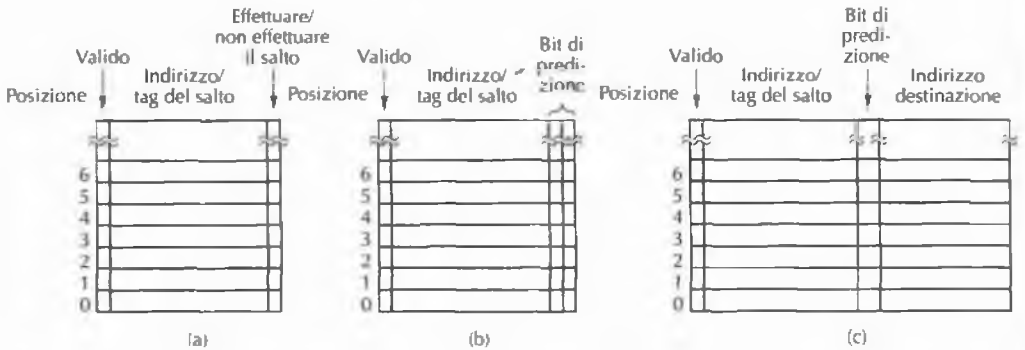
Figura 4.41 (a) Storia dei salti a 1 bit. (b) Storia dei salti a 2 bit. (c) Corrispondenza tra gli indirizzi delle istruzioni di salto e gli indirizzi destinazione.
