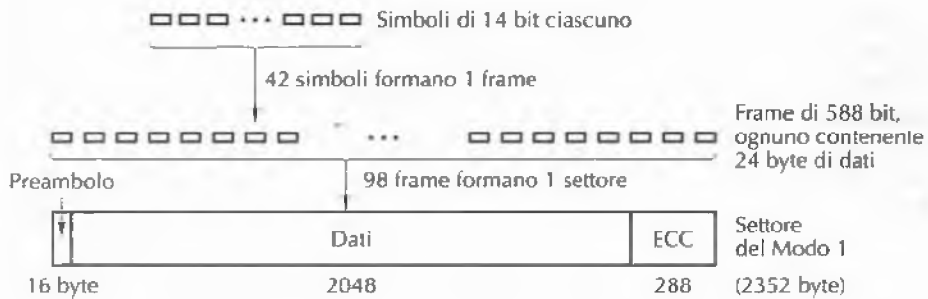
Figura 2.25 Struttura logica dei dati di un CD-ROM.
