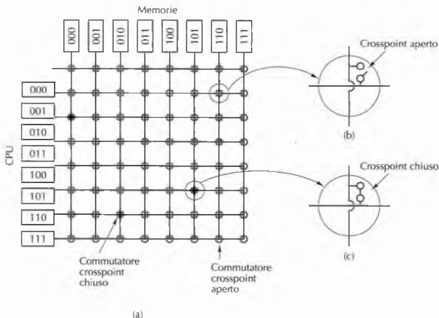
Figura 8.27 (a) Commutatore crossbar 8 x 8. (b) Crosspoint aperto. (c) Crosspoint chiuso.
