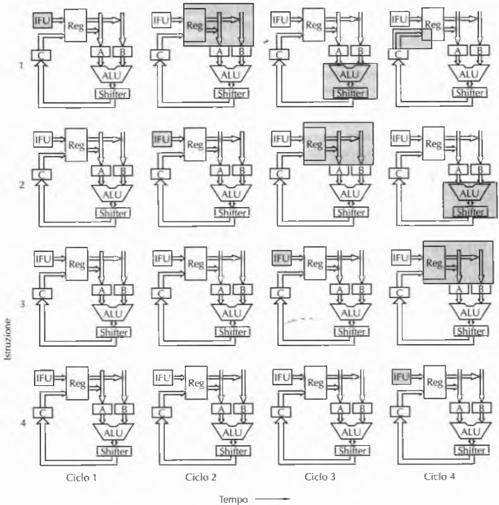
Figura 4.34 Rappresentazione grafica del funzionamento di una pipeline.
