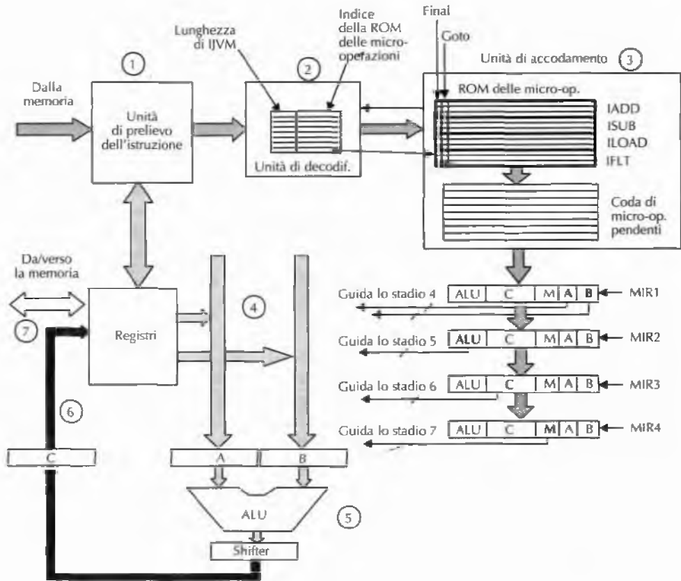
Figura 4.35 Componenti principali di Mic-4.
