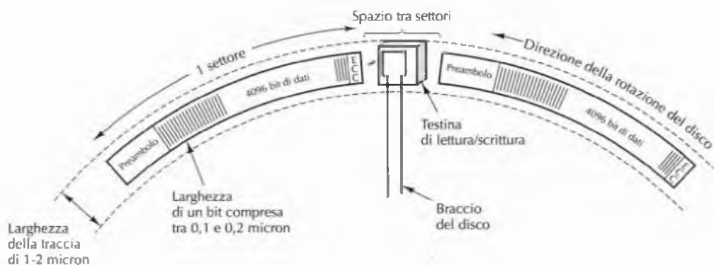
Figura 2.19 Porzione di una traccia del disco. Sono mostrati due settori.
