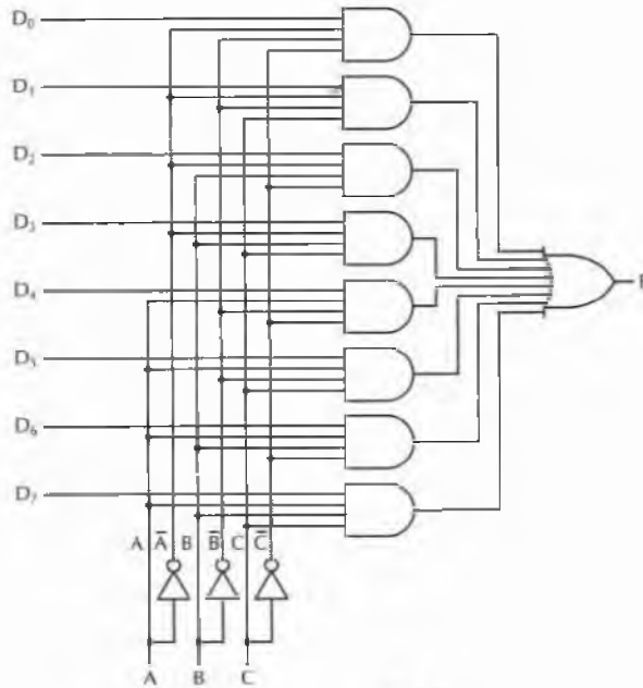
Figura 3.11 Multiplexer a otto vie.
