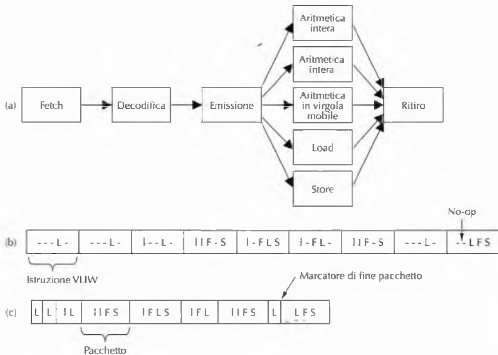
Figura 8.2 (a) Pipeline della CPU. (b) Sequenza d'istruzioni VLIW. (c) Flusso d'istruzioni con marcatori di pacchetto.
