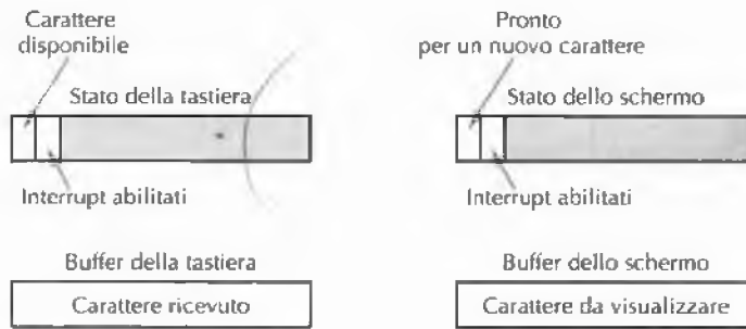
Figura 5.31 Registri dei dispositivi di un semplice terminale.
