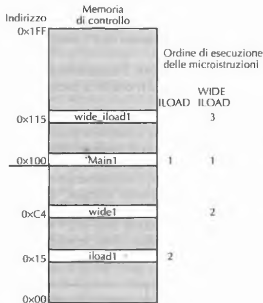
Figura 4.20 La sequenza iniziale di microistruzioni per ILOAD e WIDE ILOAD . Gli indirizzi sono puramente esemplificativi.
