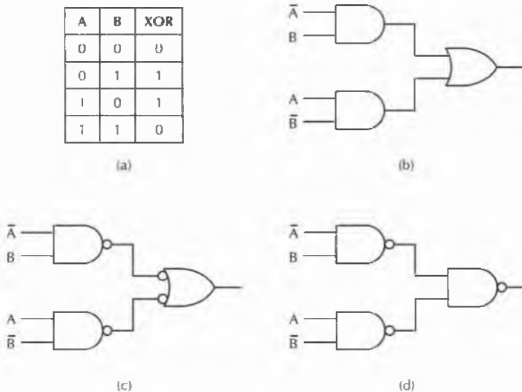
Figura 3.8 (a) Tabella di verità della funzione XOR. (b)-(d) Tre circuiti per calcolarla.
