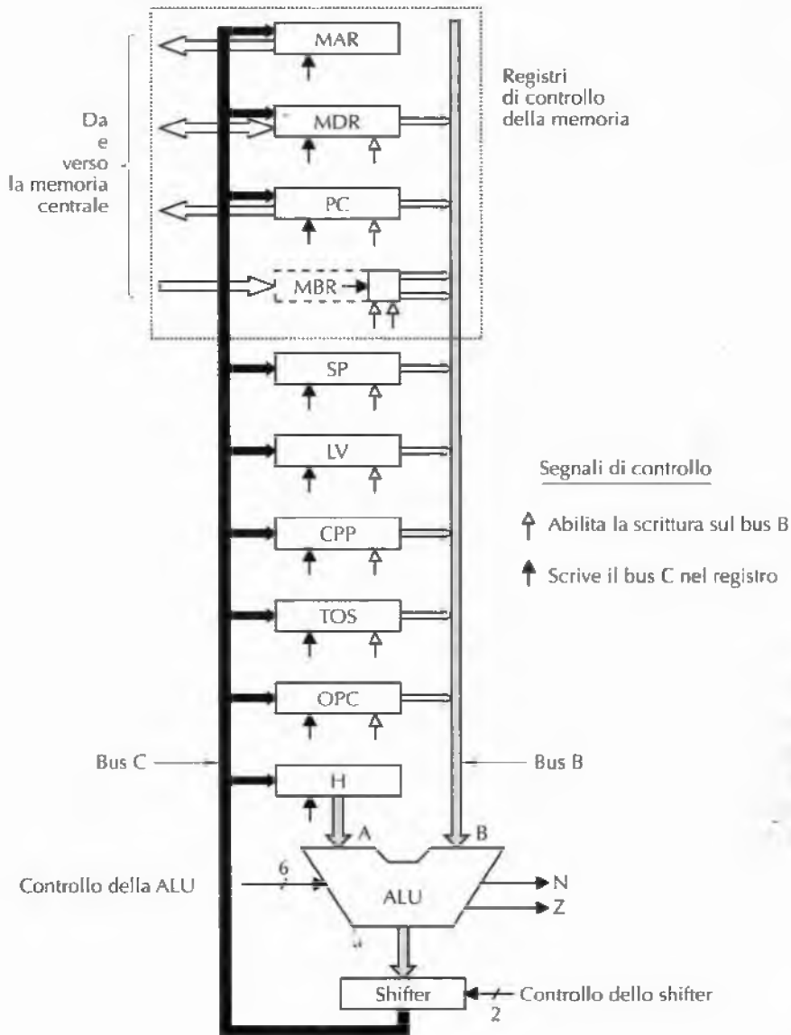
Figura 4.1 Percorso dati della microarchitettura utilizzata per l'esempio di questo capitolo.
