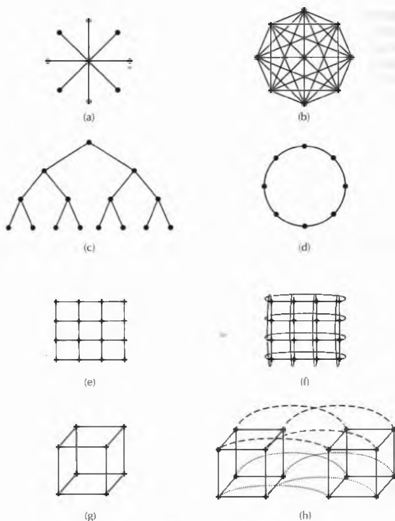
Figura 8.35 Alcune topologie. I pallini rappresentano i commutatori, mentre non sono mostrate le CPU e le memorie. (a) Stella. (b) Interconnessione completa. (c) Albero. (d) Anello. (e) Griglia. (f) Toro. (g) Cubo. (h) Ipercubo a quattro dimensioni.
