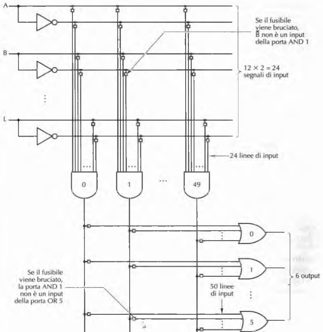
Figura 3.15 Array logico programmabile a 12 input e 6 output. I quadratini rappresentano i fusibili che possono essere bruciati per determinare la funzione da calcolare. I fusibili sono disposti in due matrici: quella superiore per le porte AND, quella inferiore per le porte OR.
