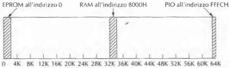
Figura 3.61 Posizione della EPROM, della RAM e del chip PIO nel nostro spazio d'indirizzamento di 64 KB.
