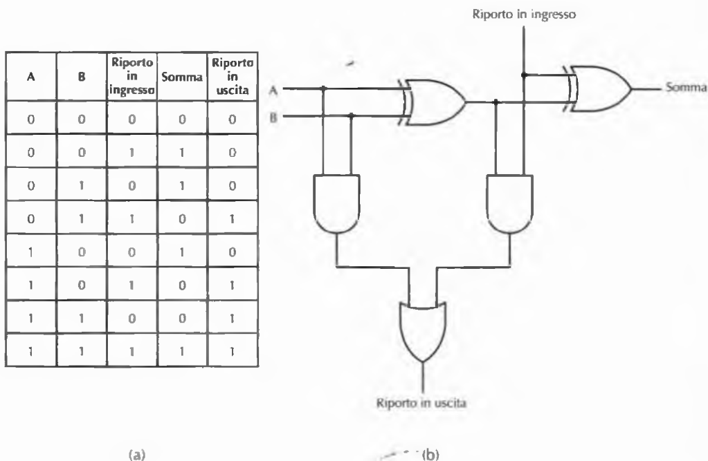
Figura 3.18 (a) Tabella di verità di un sommatore. (b) Circuito di un sommatore.
