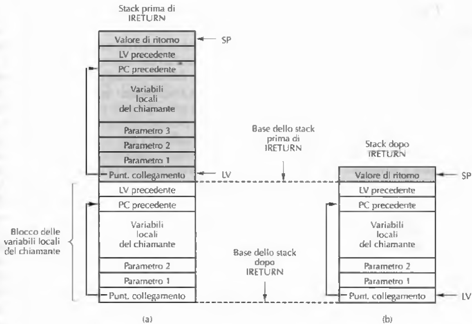
Figura 4.13 (a) Memoria prima di eseguire l'istruzione IRETURN . (b) Dopo averla eseguita.
