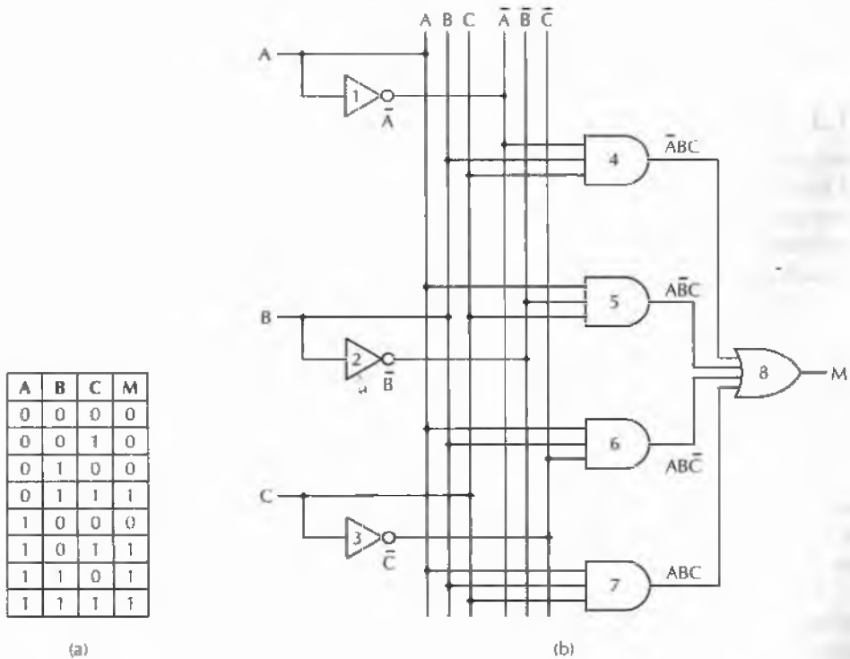
Figura 3.3 (a) Tabella di verità della funzione di maggioranza di tre variabili. (b) Un circuito per (a).
