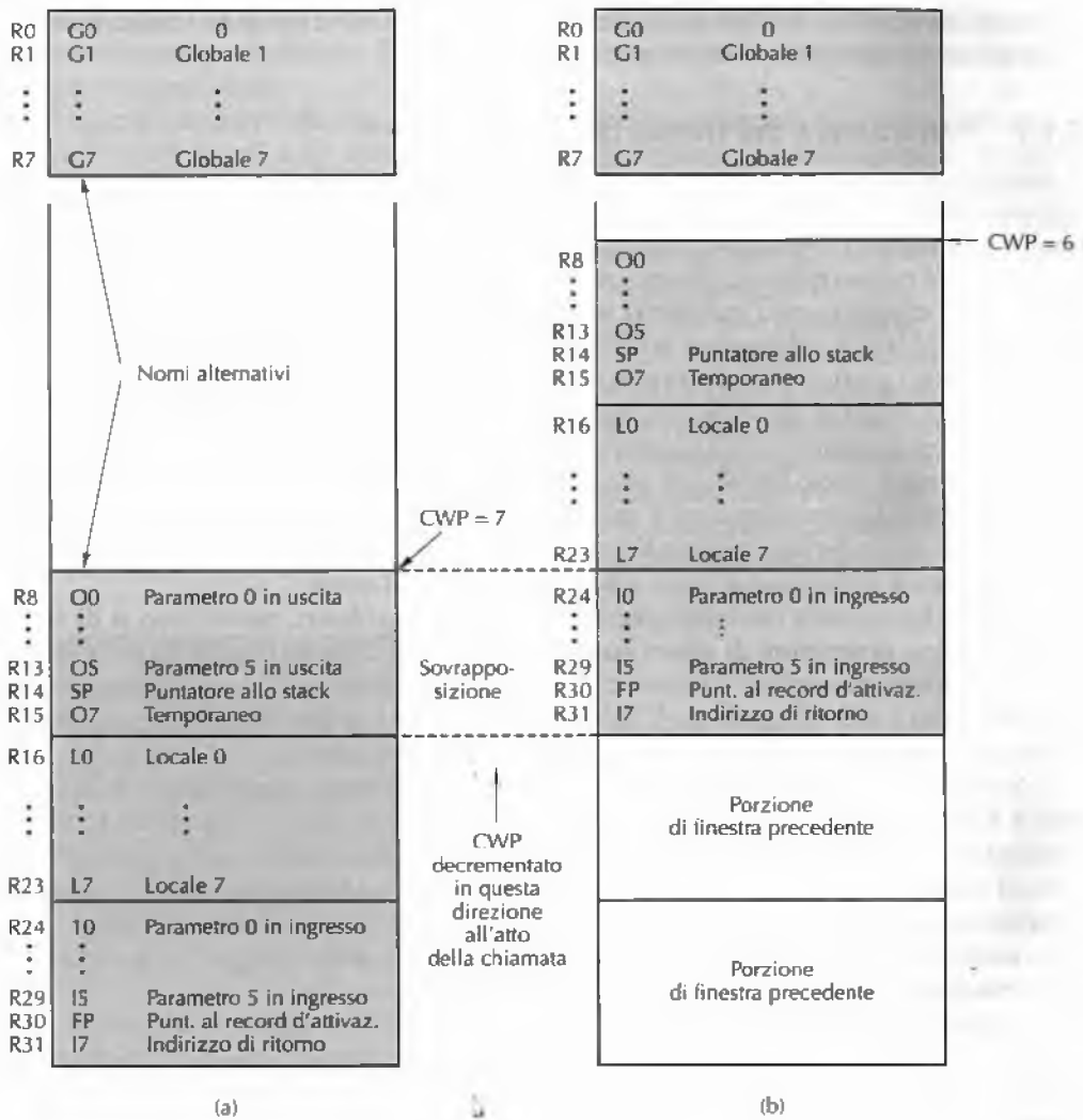
Figura 5.5 Funzionamento della finestra di registri in UltraSPARC III.
