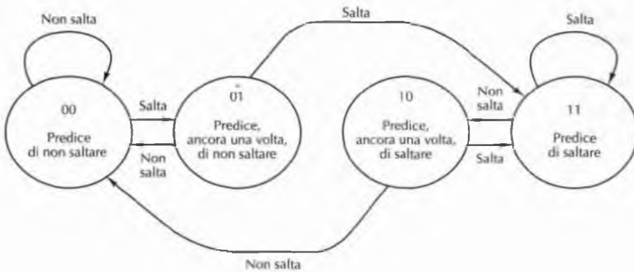
Figura 4.42 Automa a stati finiti a 2 bit per la predizione delle diramazioni.
