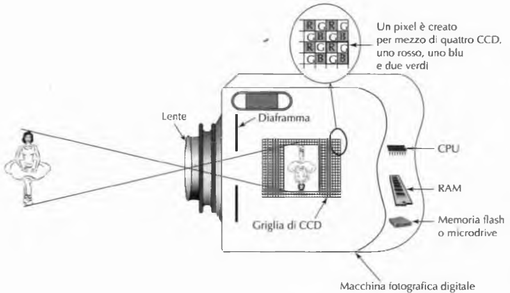
Figura 2.42 Macchina fotografica digitale.
