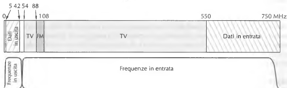
Figura 2.40 Allocazione delle frequenze in un classico sistema di TV via cavo utilizzato per l'accesso a Internet.
