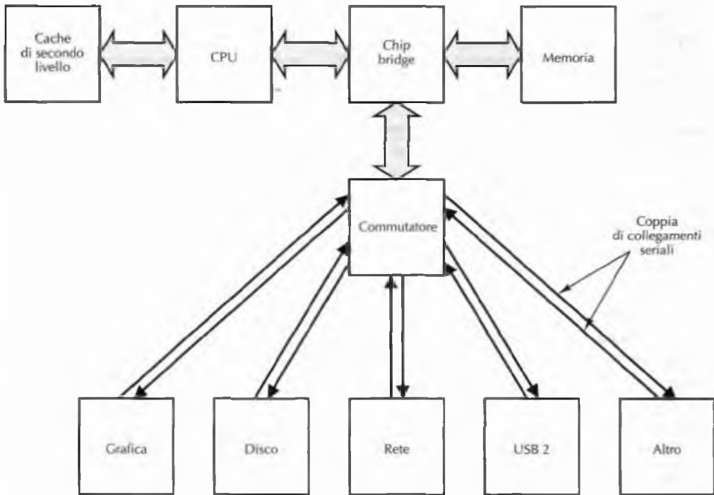
Figura 3.57 Tipico sistema PCI Express.
