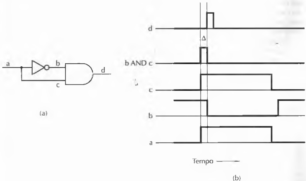
Figura 3.25 (a) Generatore d'impulsi. (b) Diagrammi temporali.
