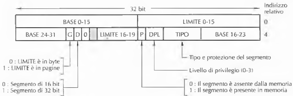
Figura 6.13 Descrittore di un segmento di codice nel Pentium 4. I segmenti di dati sono leggermente diversi.
