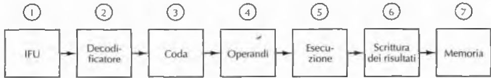
Figura 4.36 Pipeline di Mic-4.
