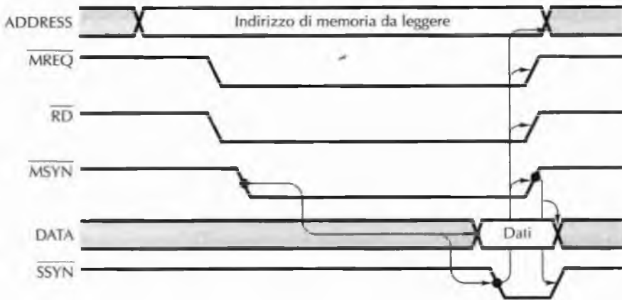
Figura 3.39 Funzionamento di un bus asincrono.
