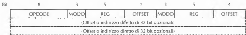
Figura 5.26 Semplice progetto dei formati d'istruzione di una macchina a due indirizzi.
