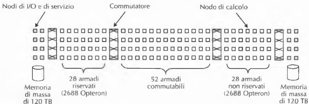
Figura 8.39 Visione dall'alto di Red Storm.
