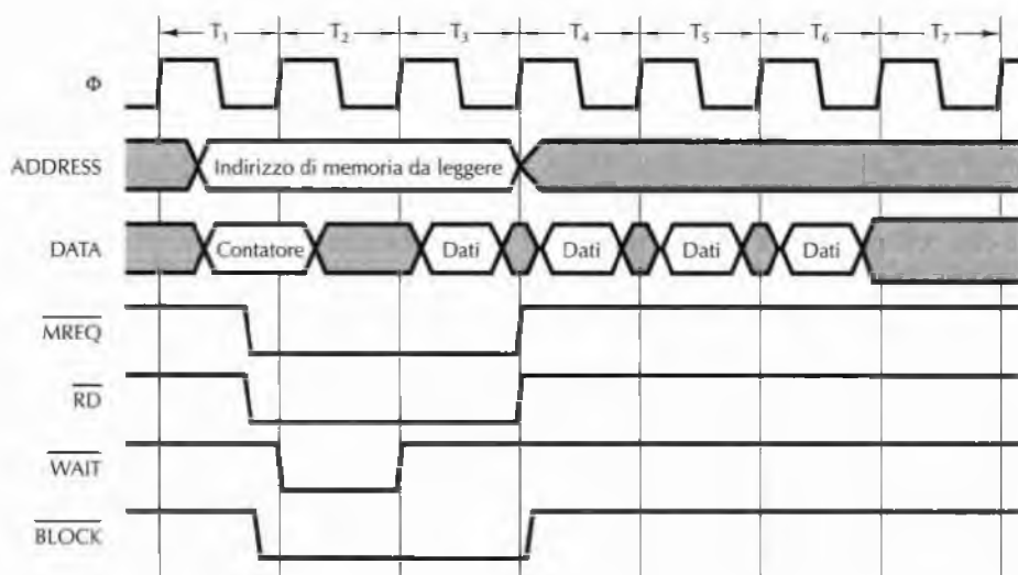
Figura 3.42 Trasferimento di un blocco.
