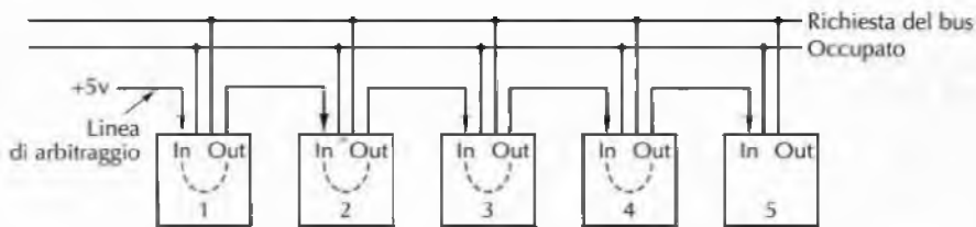
Figura 3.41 Arbitraggio decentralizzato del bus.
