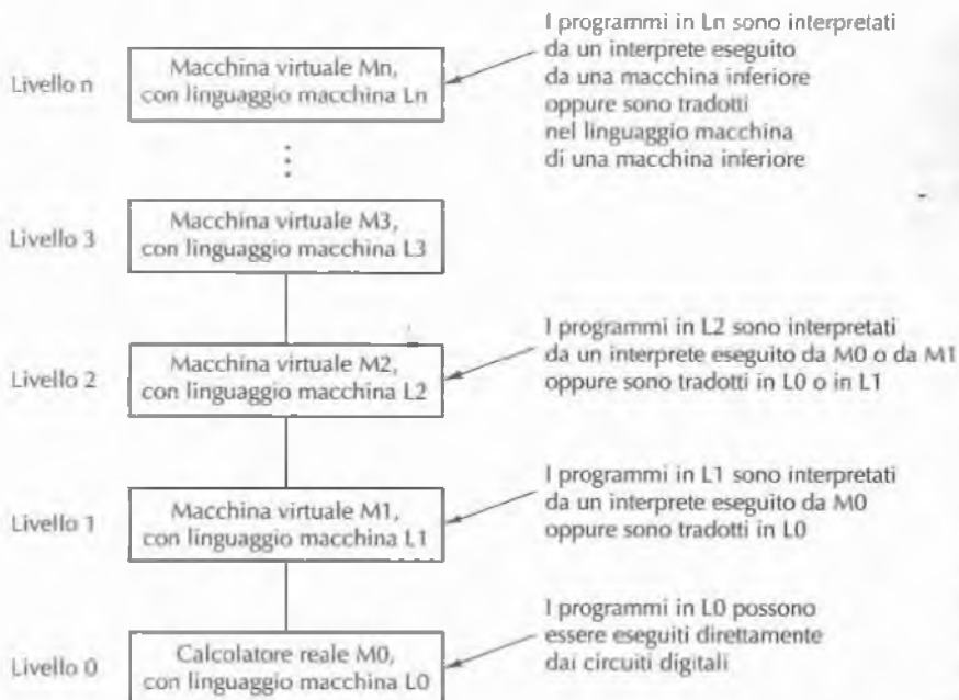
Figura 1.1 Macchina multilivello.
