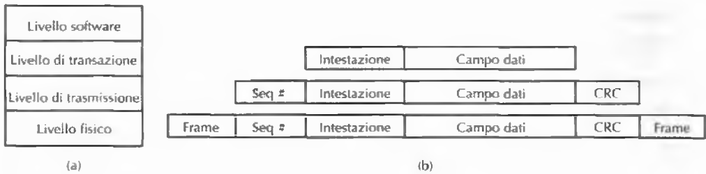
Figura 3.58 (a) Pila di protocolli di PCI Express. (b) Formato di un pacchetto.
