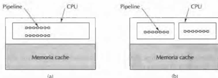
Figura 8.10 Multiprocessori a singolo chip. (a) Un chip con pipeline duplice. (b) Un chip con due core.
