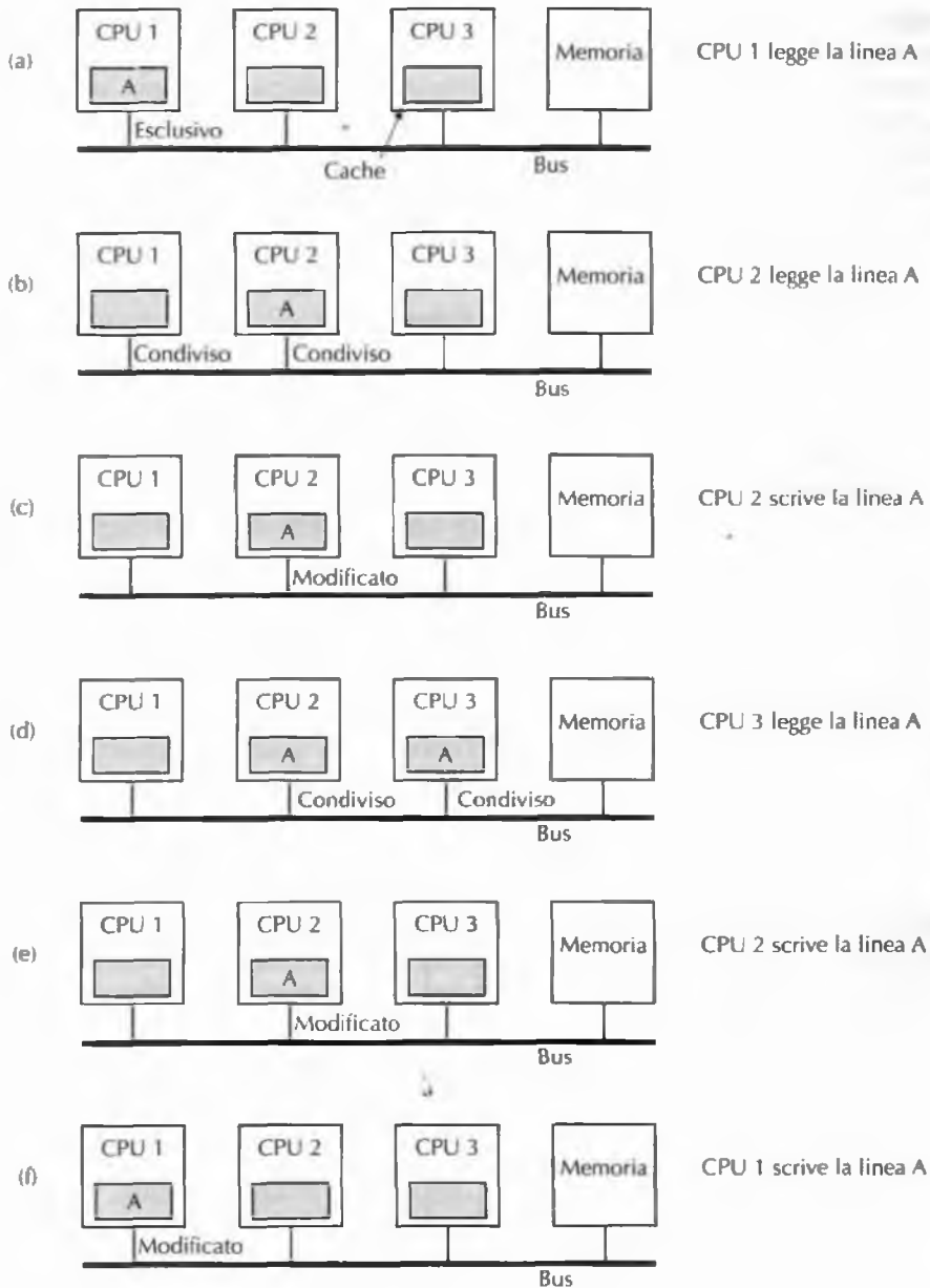
Figura 8.26 Protocollo MESI di coerenza delle cache.
