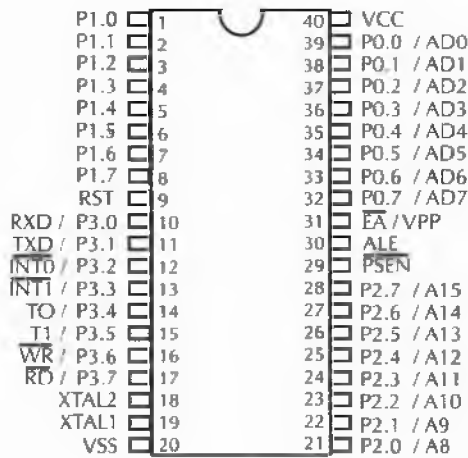
Figura 3.49 Disposizione fisica dei contatti dell'8051.
