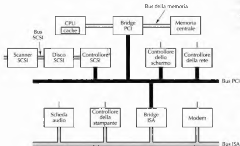
Figura 2.30 Tipico PC odierno con un bus PCI e un bus ISA. La scheda audio e il modem sono dispositivi ISA; il controllore SCSi è un dispositivo PCI.
