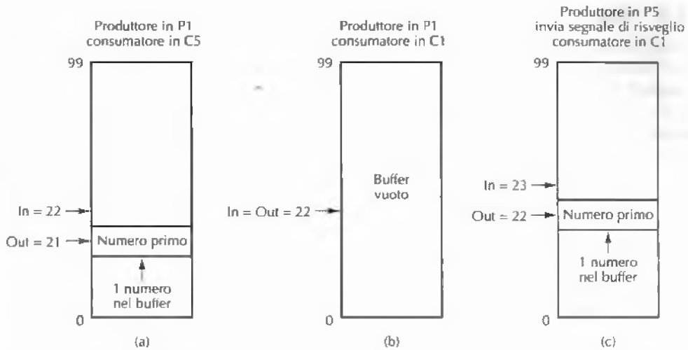
Figura 6.26 Insuccesso del meccanismo di comunicazione tra produttore e consumatore.
