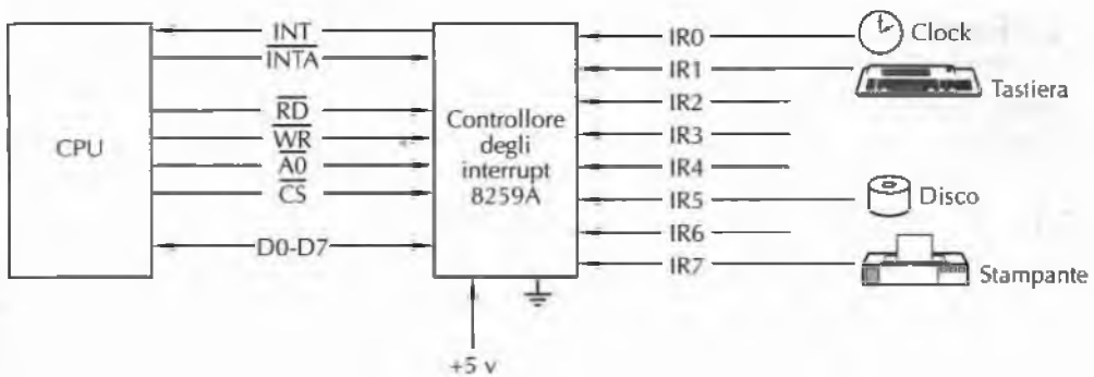
Figura 3.43 Utilizzo del controllore degli interrupt 8259A.
